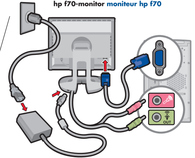
hp f70-monitor moniteur hp f70
