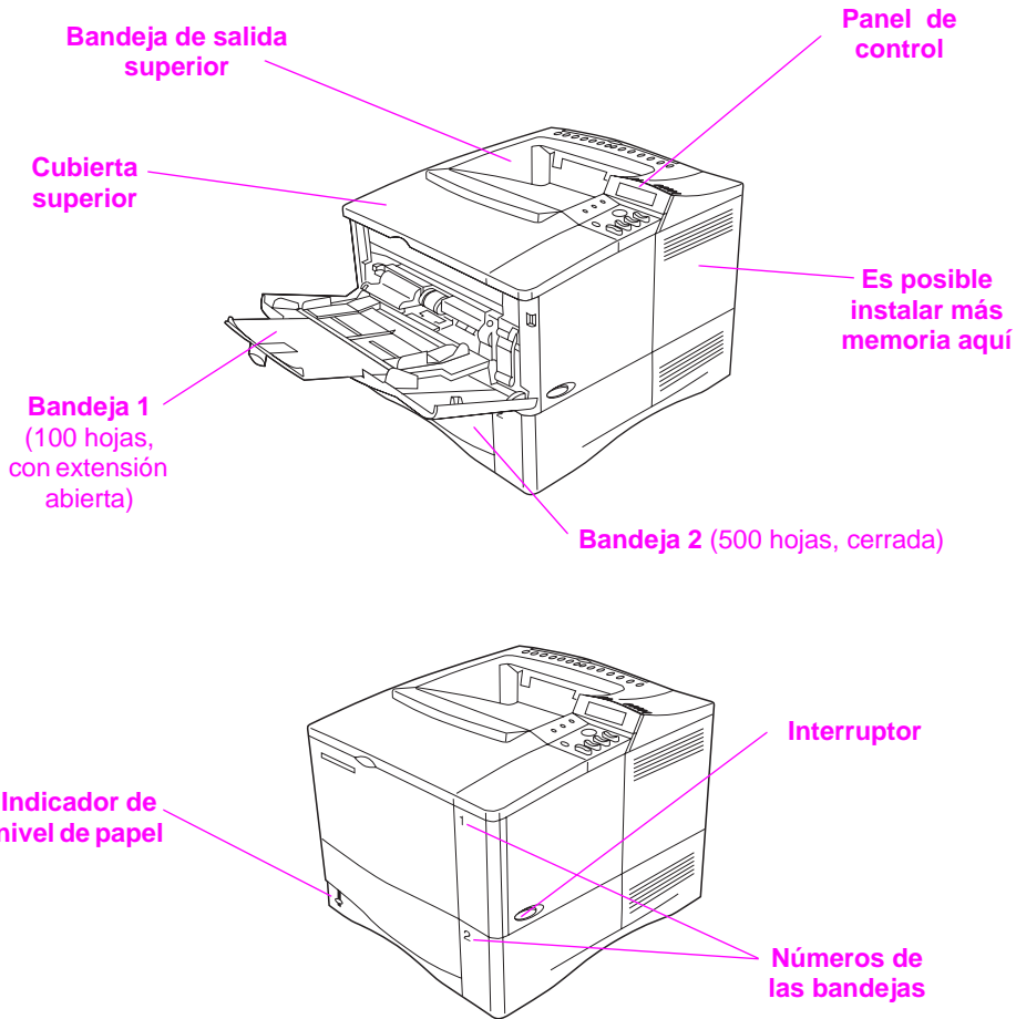
Figura 3 Componentes de la impresora (vista frontal)
