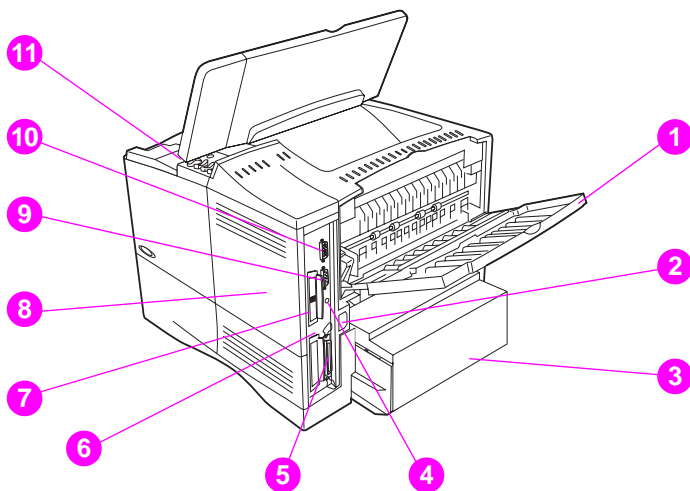
Figura 4 Componentes de la impresora (vista posterior)
