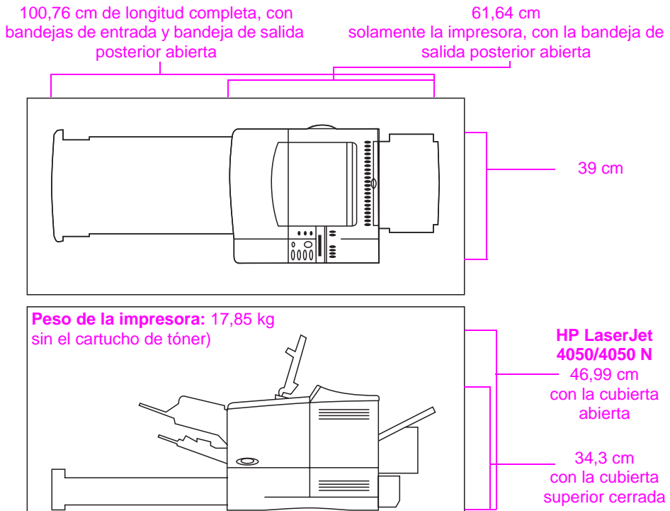
Figura 2 Dimensiones de la impresora
