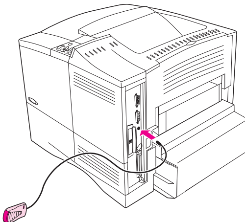
Kuva 8 HP LaserJet 4050 N -kirjoittimen infrapunaportti
