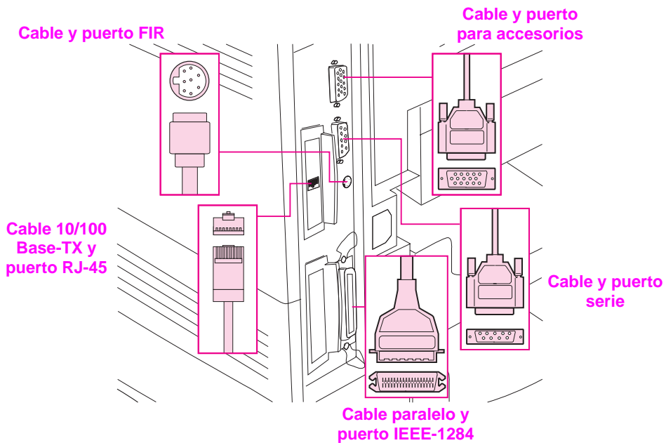
Figura 7 Puertos de interfaz
