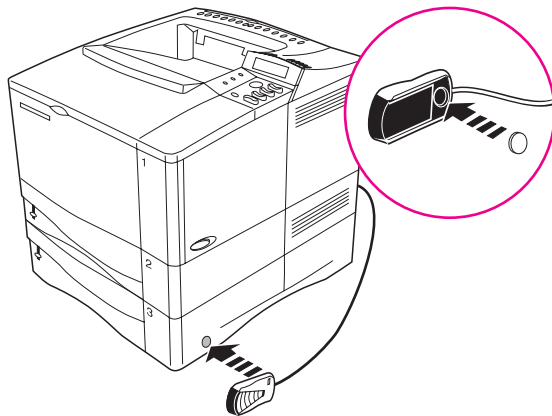
Figura 9 Adhesión de los cierres de Velcro
