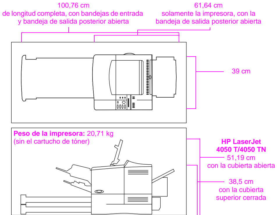
Figura 2 Dimensiones de la impresora
