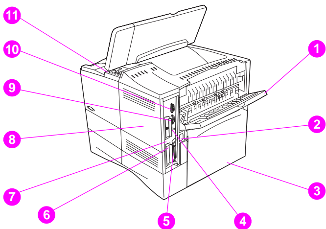
Figura 4 Componentes de la impresora (vista posterior)
