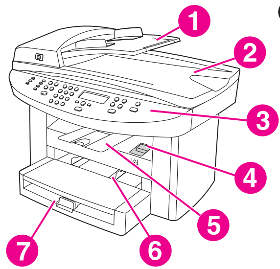
איתור חלקי המכשיר. 1 מגש ההזנה של ADF; 2 מכסה הסרוק השטוח; וסל הפלט של ADF; 3 לוח בקרה; 4 תפס שחרור דלת מחסנית ההדפסה; 5 סל פלט; 6 מגש הזנה מועדף; 7 מגש הזנת חומרי הדפסה;
