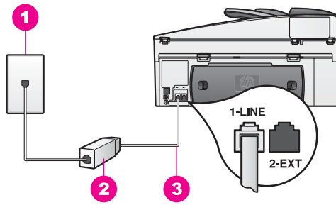
מראה אחורי של HP all-in-one
