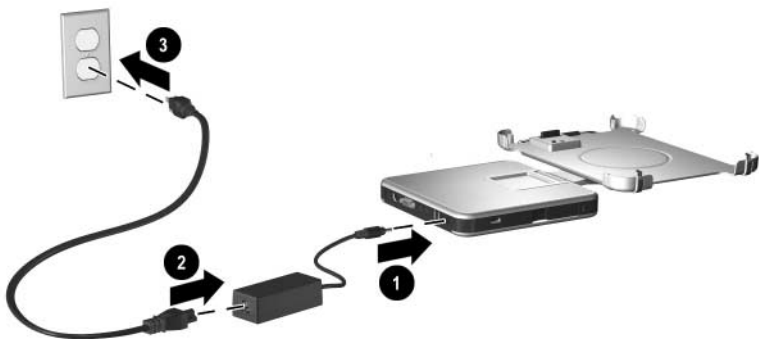
Aansluiten op een voedingsbron
