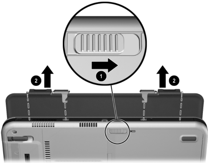
Schermbeschermer losmaken van de tablet-pc
