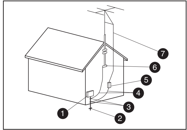
안테나 접지
