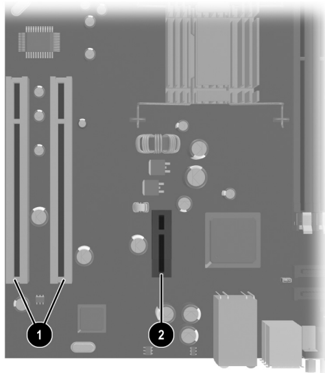
Emplacement des supports pour carte d'extension
