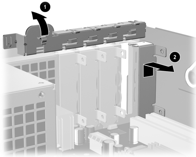
Retrait de l'obturateur du support d'extension
