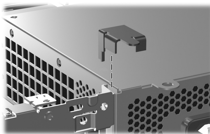
Installation du clip de sécurité
