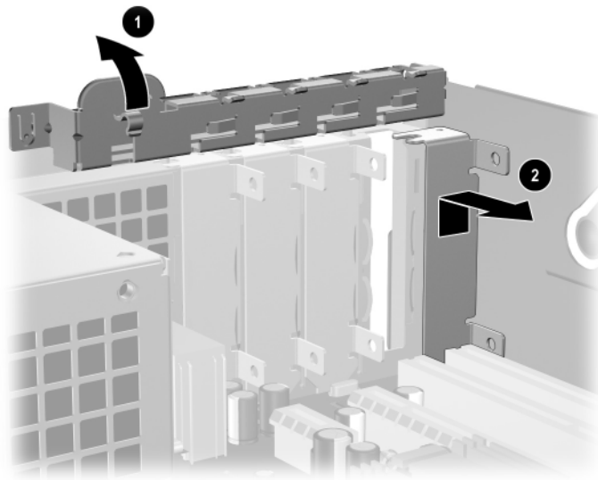
Entfernen der Abdeckung eines Erweiterungssteckplatzes
