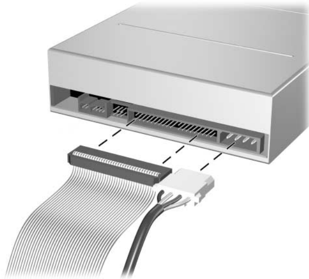
Anschließen der Strom- und Datenkabel
