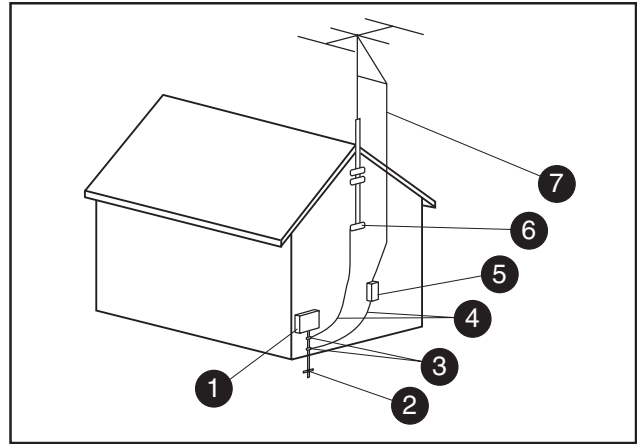
안테나 접지
