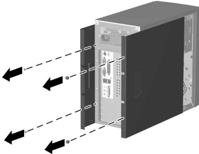
Retrait des panneaux d'accès
