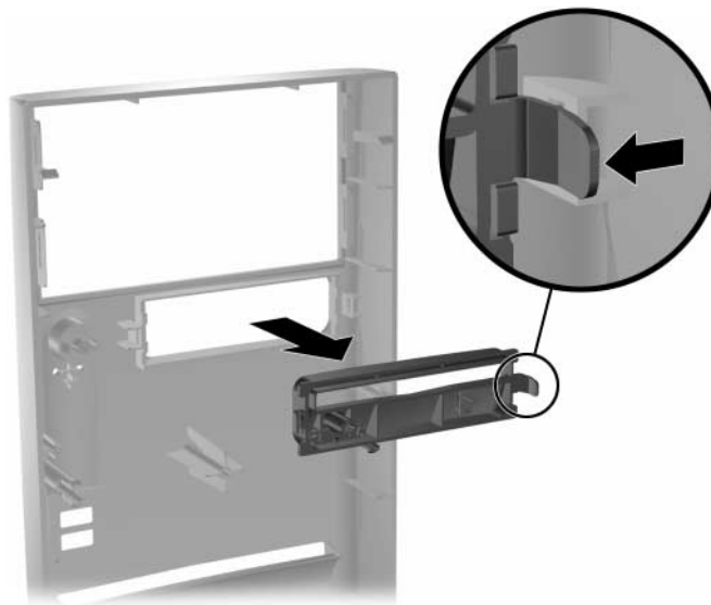
Retrait du cache protecteur
