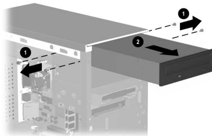
Retrait d'une unité de 5,25 pouces
