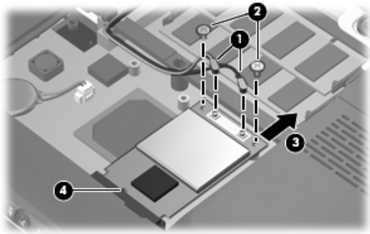
Removing a Mini Card Module
