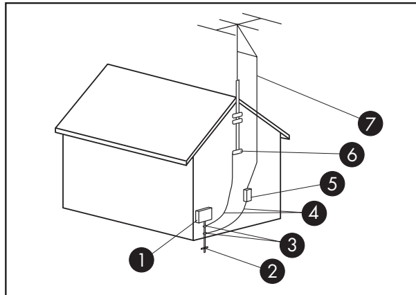
Antennenerdung
