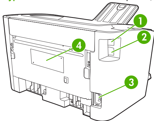
Сурет 1-4 HP LaserJet P1500 Сериялы, артқы көрінісі (HP LaserJet P1505n көрсетілген)
