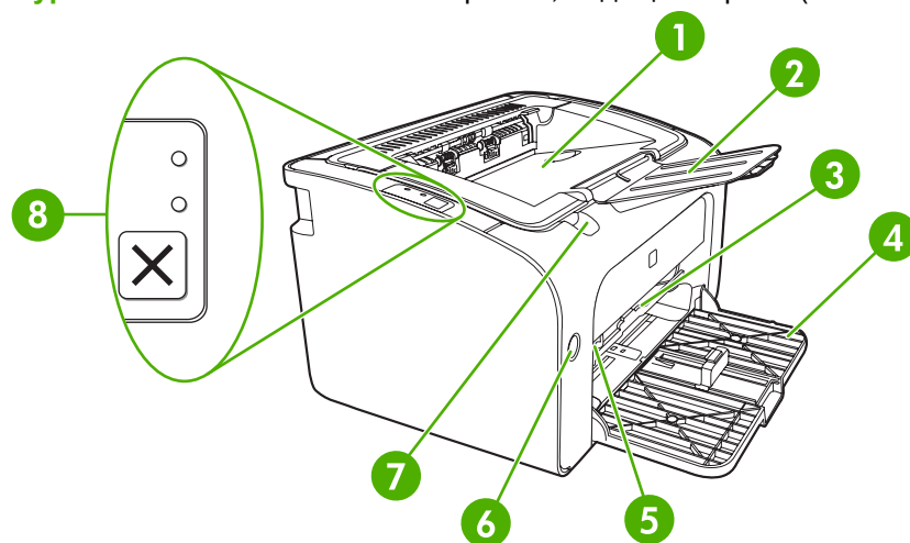
Сурет 1-1 HP LaserJet P1000 Сериялы, алдыңғы көрінісі (HP LaserJet P1006/P1009 көрсетілген)
