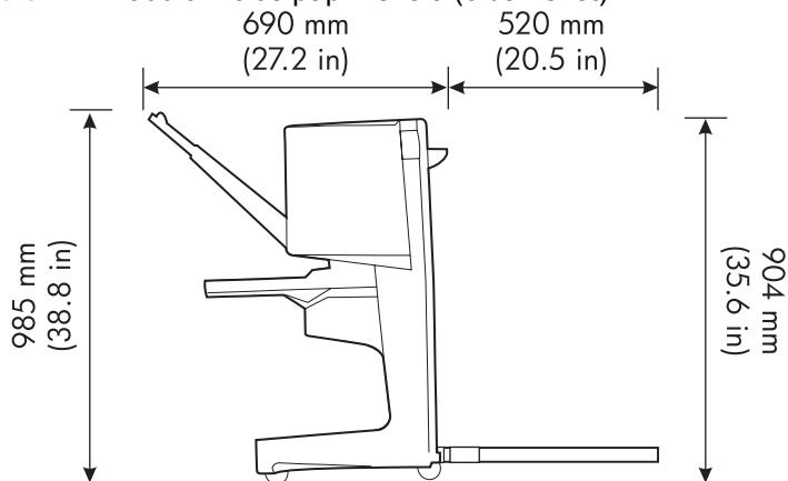
A-1 ábra HP Többfunkciós papírkezelő (oldalnézet)
