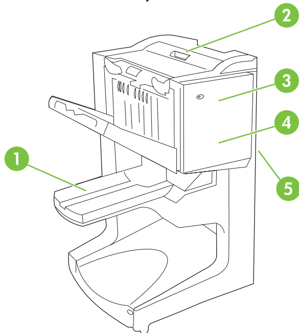
3-1 ábra Elakadási helyek
