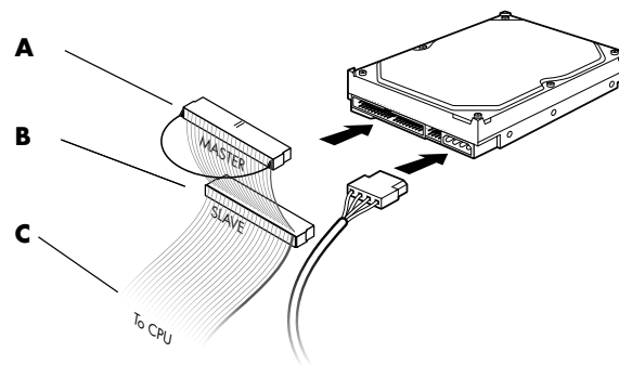
Paralleles ATA-Laufwerk
