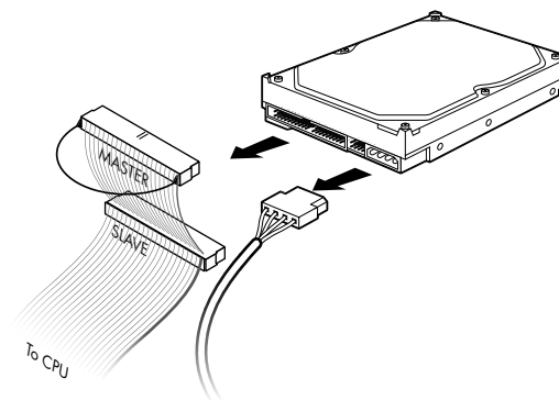
Paralleles ATA-Laufwerk
