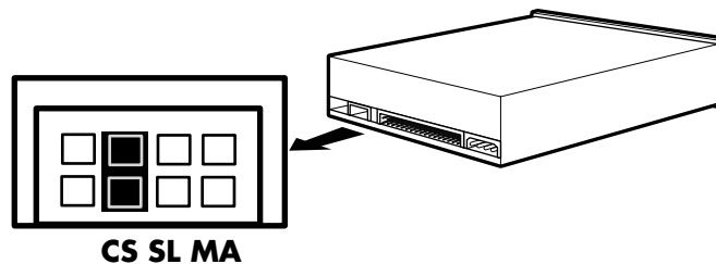
Cable-Select-Steckbrücke
