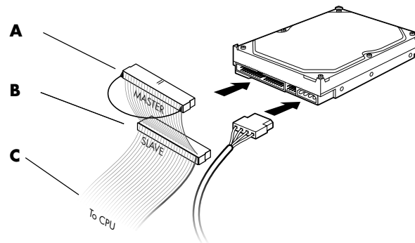
Paralleles ATA-Laufwerk
