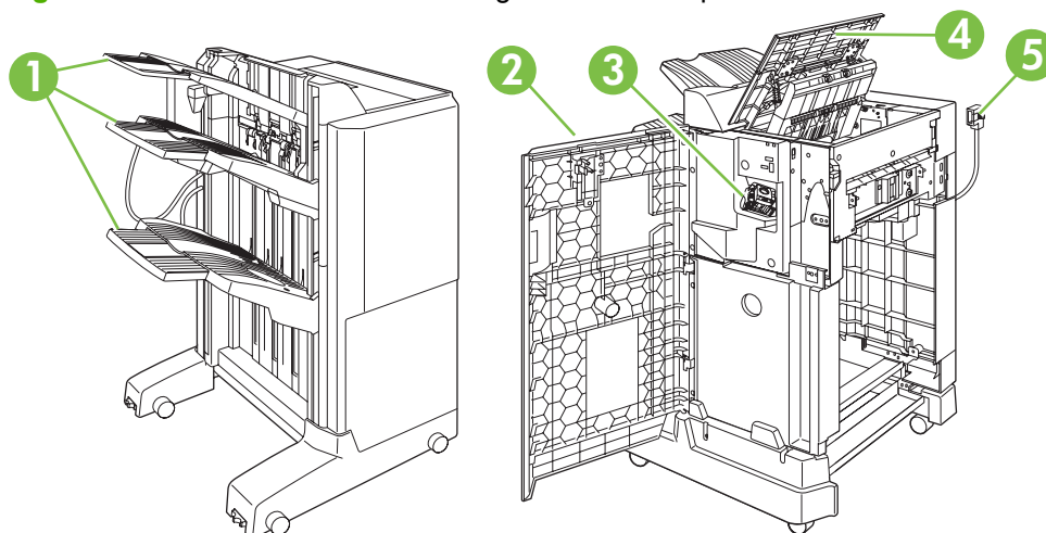
Figura 7-1 Accessorio cucitrice/raccogliitore a 3 scomparti
