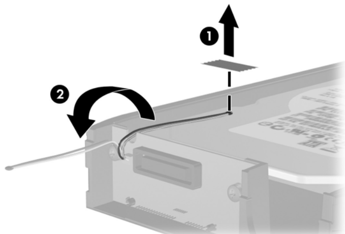
図 2-42 温度センサの取り外し
