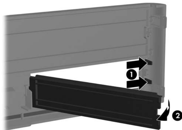
図 2-4 3.5 インチ ドライブ ベイ カバーの取り外し
