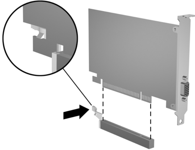
図 2-15 PCI Express x16 拡張カードの取り外し
