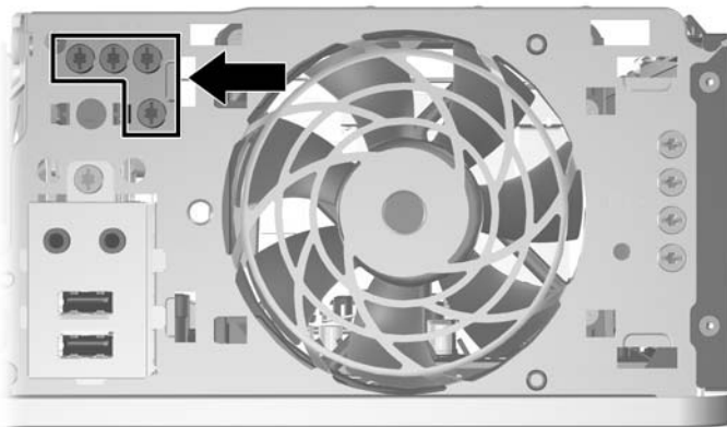
図 2-19 セカンダリ ハードディスク ドライブ用 6-32 インチネジの位置
