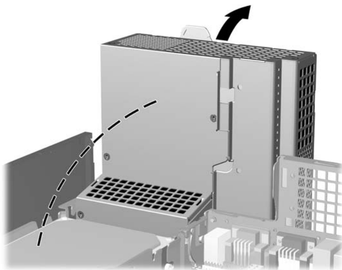
図 2-36 電源供給装置の持ち上げ
