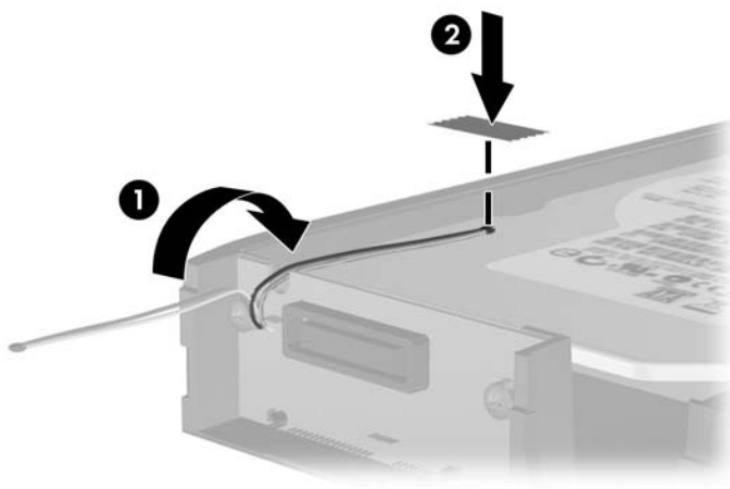
図 2-47 温度センサの再取り付け
