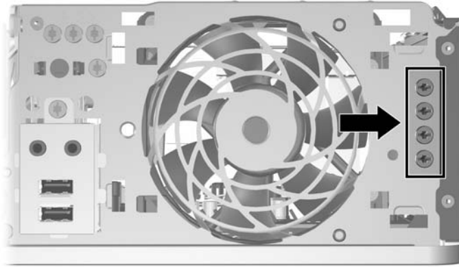
図 2-20 オプティカル ドライブ用の予備のガイド用 M3 ネジの位置
