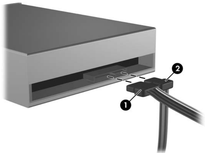
図 2-23 電源ケーブルとデータ ケーブルの取り外し
