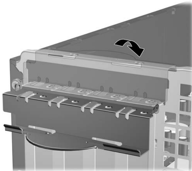
図 2-17 拡張スロットの固定ラッチを閉じる
