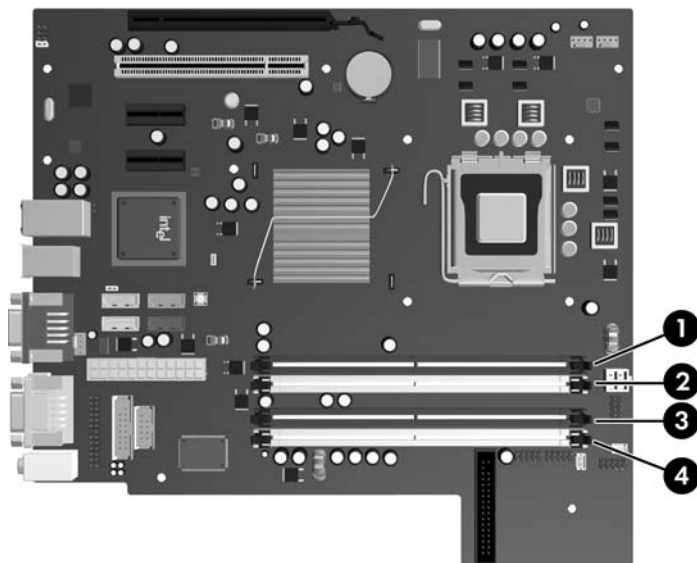
図 2-9 DIMM ソケットの位置
