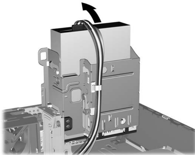
図 2-22 ドライブ ケージを上回転させる
