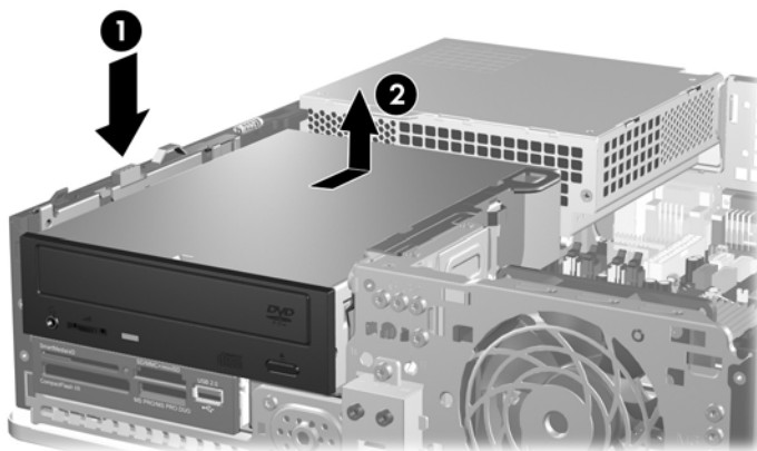
図 2-25 オプティカルドライブの取り外し
