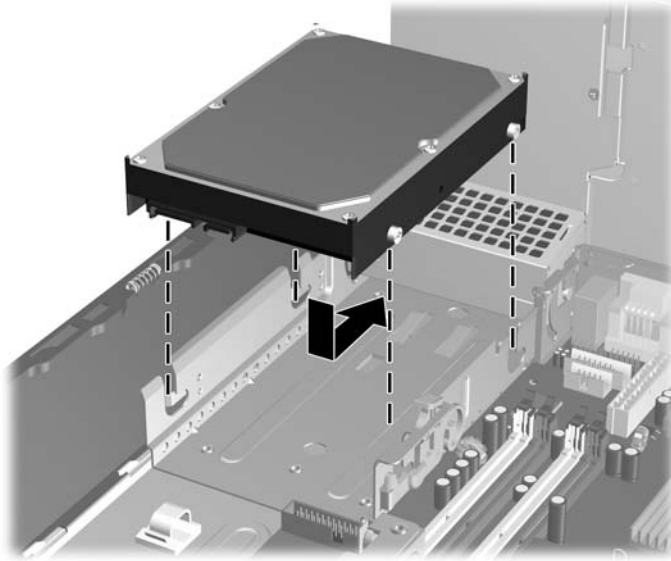
図 2-40 ハードディスク ドライブの取り付け
