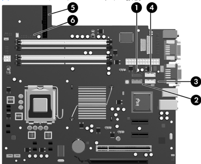
図 2-21 システムボードのドライブ接続
