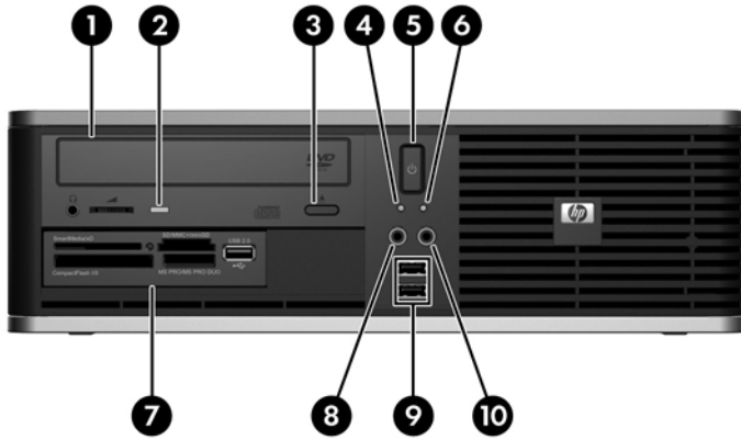
図 1-2 フロント パネルの各部
