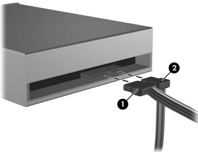
図 2-29 電源ケーブルとデータ ケーブルの接続
