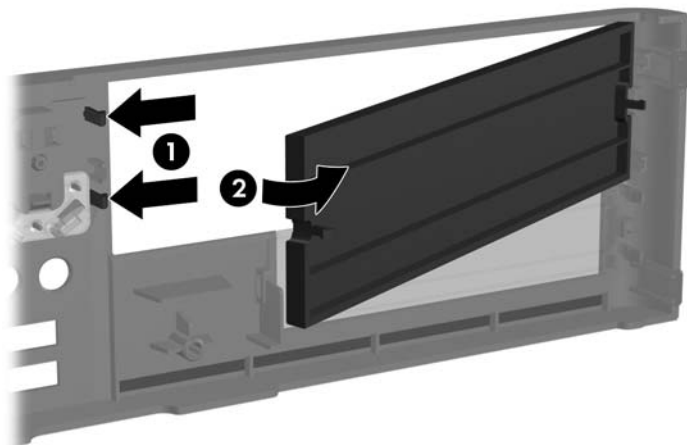
図 2-5 5.25 インチ ドライブ ベイ カバーの取り外し
