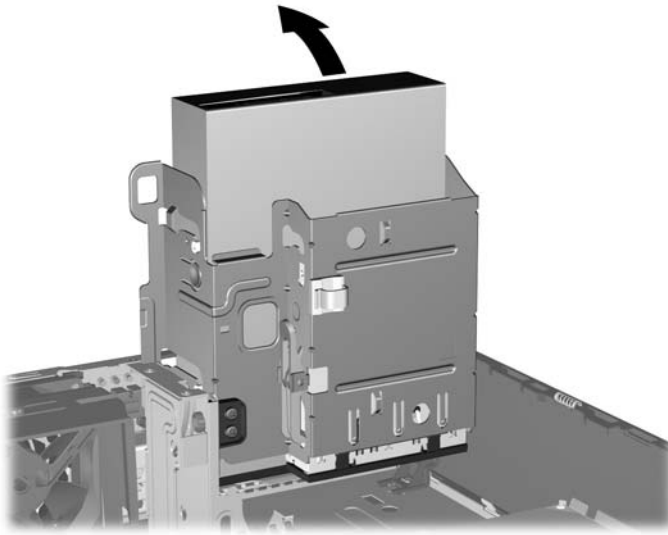
図 2-28 ドライブ ケージを上回転させる
