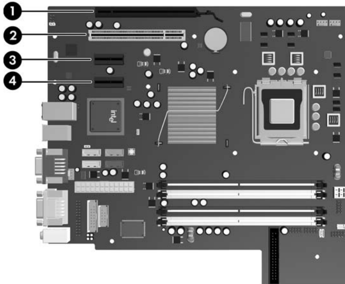
図 2-11 拡張スロットの位置
