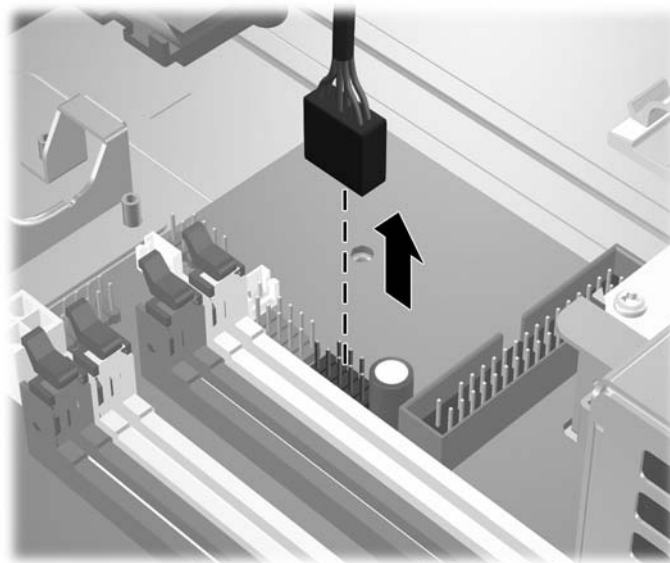
図 2-32 メディア カード リーダー ケーブルの取り外し
