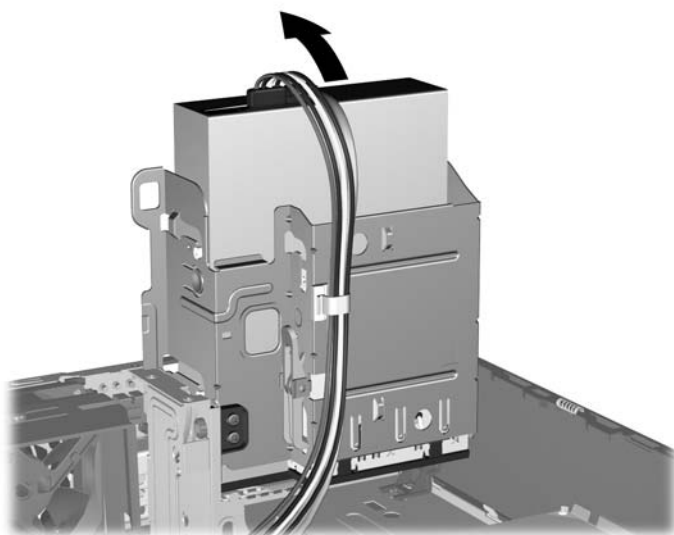
図 2-35 ドライブ ケージを上回転させる
