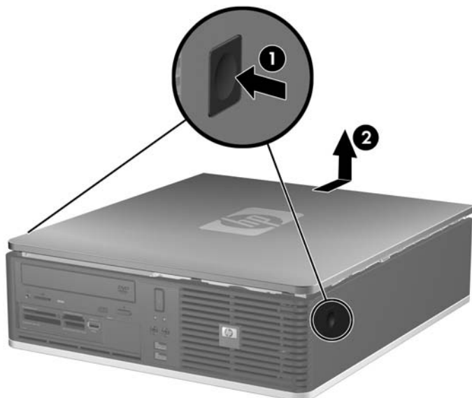
図 2-1 アクセス パネルの取り外し
