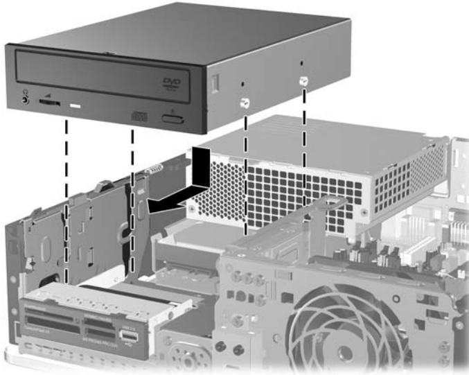
図 2-27 オプティカルドライブの取り付け
