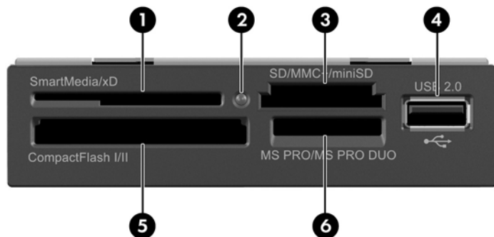
図 1-3 メディアカードリーダーの各部
