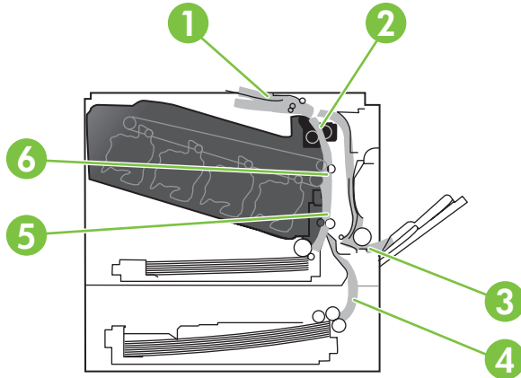
그림 11-1 용지 걸림 위치
