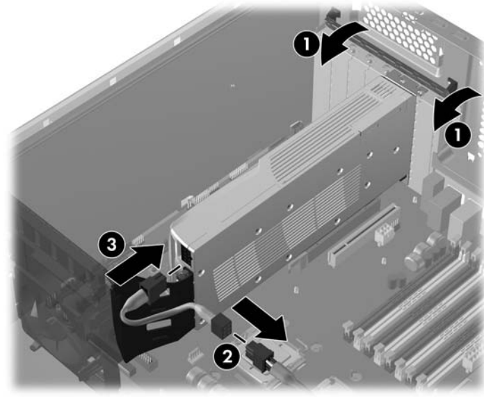
図 6 電源アダプタ ケーブルの取り付け
