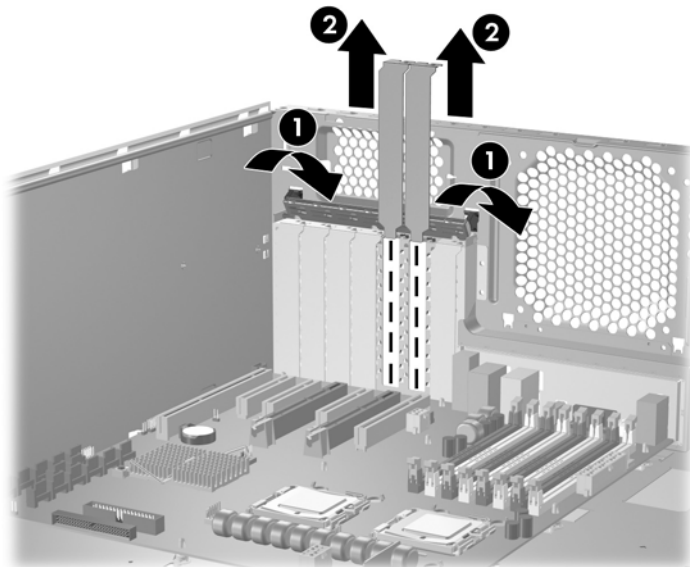
図 4 保持レバーの解放とスロット カバーの 取り外 し
