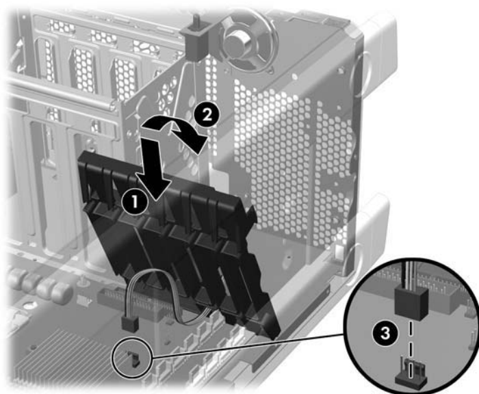
図3 シャーシへの前面ファン/カードガイドアセンブリの取り付け
