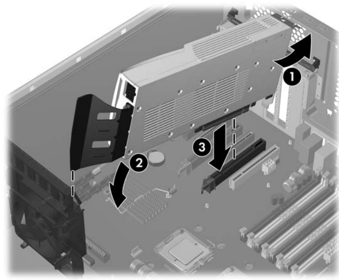
図 5 FX5800 グラフィックス カードの位置合わせおよび取り付け
