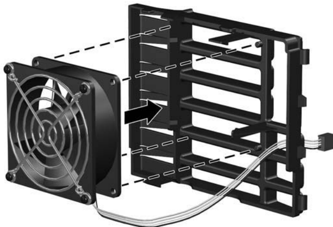
図2 カードガイドへの前面ファンの取り付け
