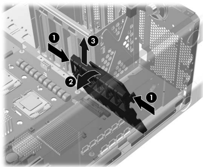
図 1 シャーシからのカード ガイドの取り外し
