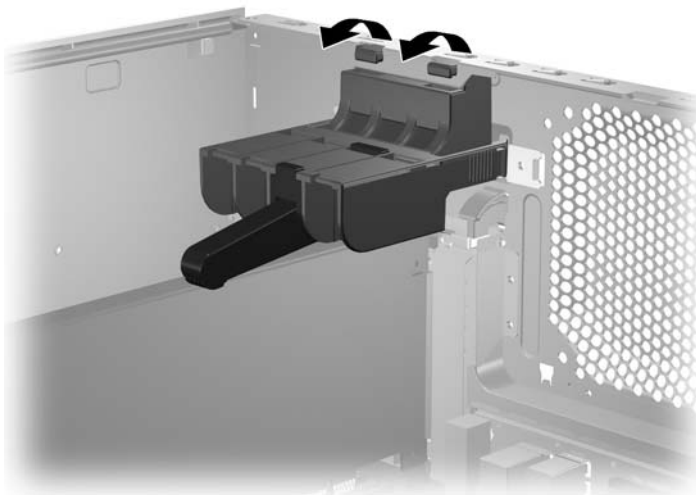
図 7 カード サポート ブラケットの取り付け
