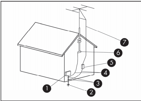
天線接地
