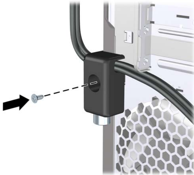
Obrázok 37 Pripojenie zámku k šasi
