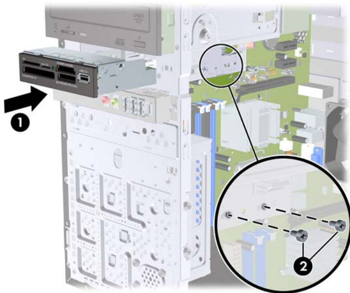
Obrázok 20 Inštalácia 3,5-palcového zariadenia (zobrazený je čítač mediálnych kariet)
