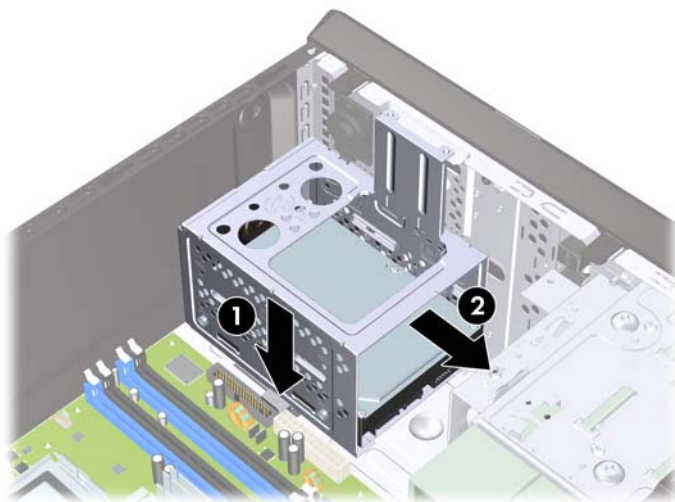
Obrázok 22 Uvoľnenie šachty pevného disku
