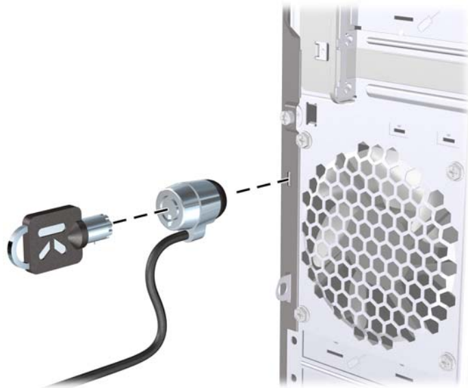
Obrázok 33 Inštalácia lankového zámku
