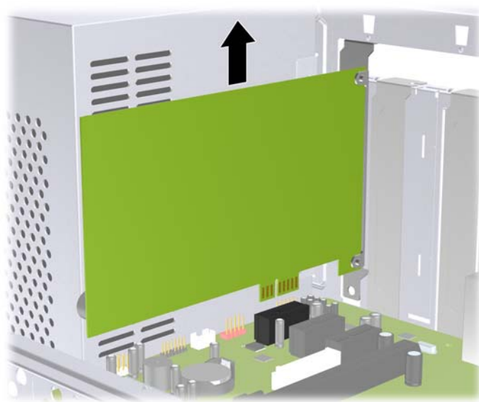
Obrázok 9 Vybratie rozširujúcej karty PCI Express x1
