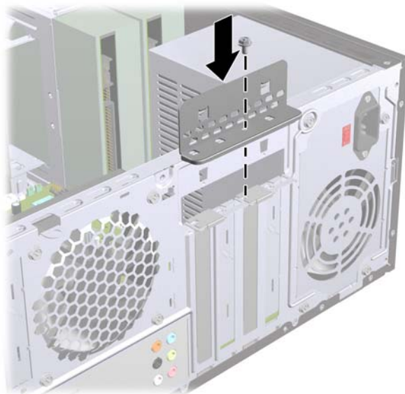
Obrázok 12 Pripevnenie rozširujúcich kariet a krytov umiestnených na zásuvkách
