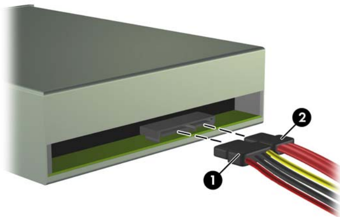
Obrázok 15 Odpojenie napájacieho a dátového kábla
