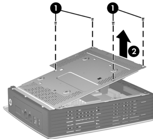
Figure 2-4 Retrait du cache métallique latéral
