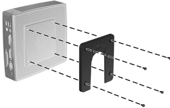
Figure C-2 Montage de HP Quick Release sur le client léger
