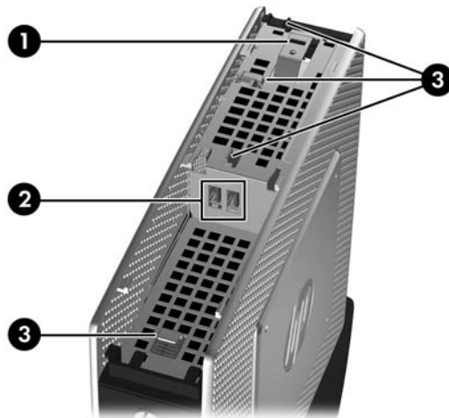
Figure 1-3 Éléments du panneau supérieur, vue interne
