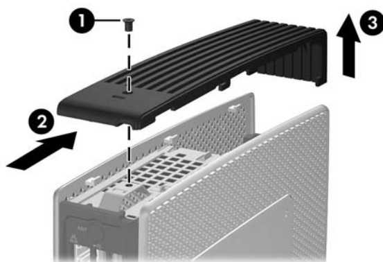
Figure 2-1 Retrait du cache du compartiment USB sécurisé
