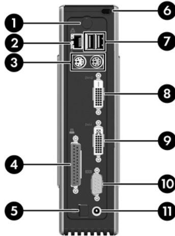
Figure 1-4 Éléments du panneau arrière
