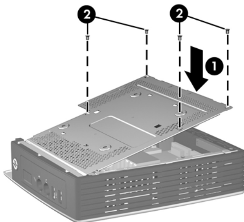
Figure 2-5 Remise en place du cache métallique latéral
