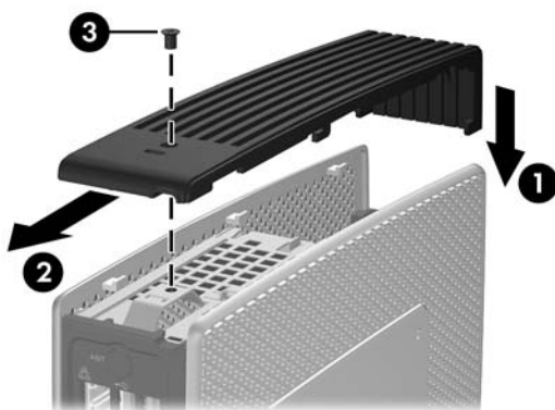
Figure 2-2 Remise en place du cache du compartiment sécurisé
