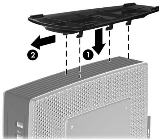
Afbeelding 1-7 Standaard installeren
