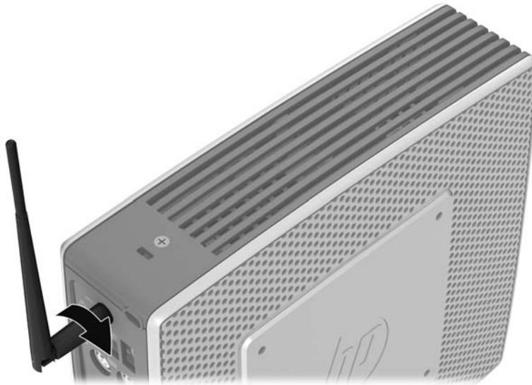
Afbeelding 1-5 Antenne installeren
