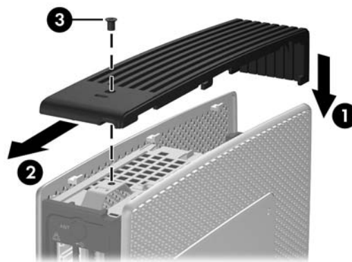
Afbeelding 2-2 Afdekplaatje van het beveiligde USB-compartiment terugplaatsen
