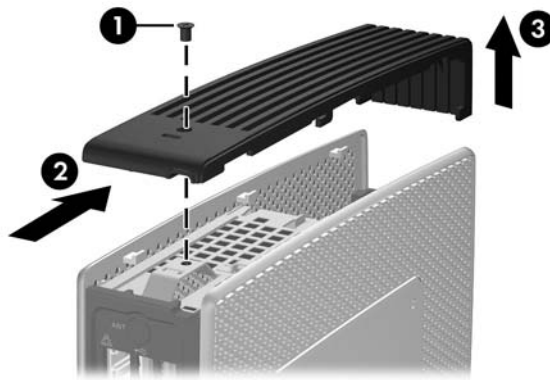
Afbeelding 2-1 Afdekplaatje van beveiligd USB-compartiment verwijderen
