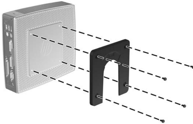
Afbeelding C-2 HP Quick Release aansluiten op de thin client
