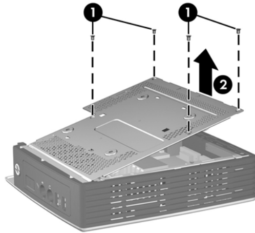
Afbeelding 2-4 Metalen zijpaneel verwijderen
