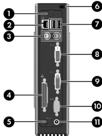
Afbeelding 1-4 Onderdelen op het achterpaneel
