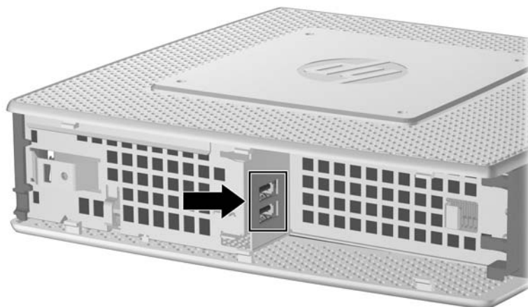
圖示 2-6 安全 USB 區間的 USB 連接埠
