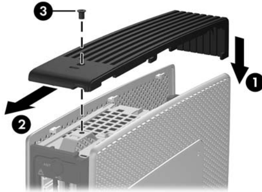
圖示 2-2 裝回安全區間外殼
