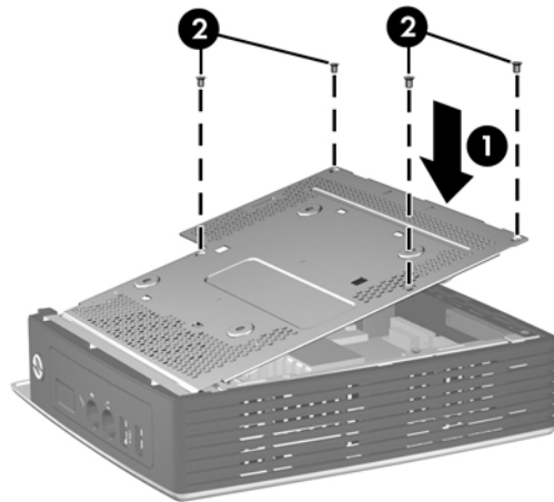
圖示 2-5 裝回金屬側面外殼
