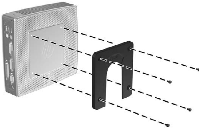
圖示 C-2 將 HP 快速釋放連接到精簡型電腦
