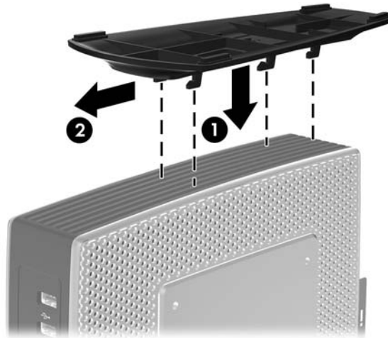
圖示 1-7 安裝機座
