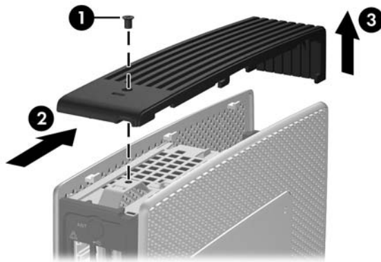
圖示 2-1 拆下安全 USB 區間外殼
