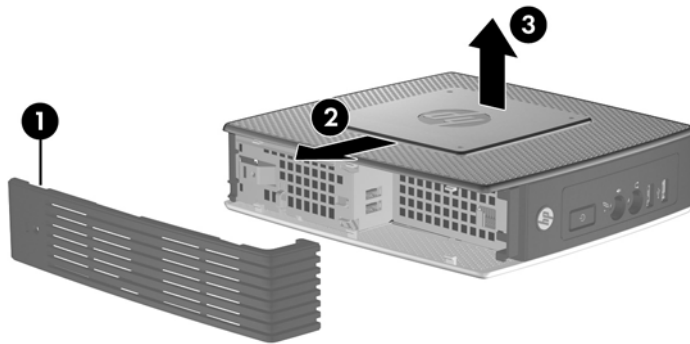
圖示 2-3 拆下側面存取面板
