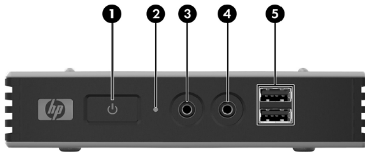
Afbeelding 2-1 Onderdelen op het frontpaneel
