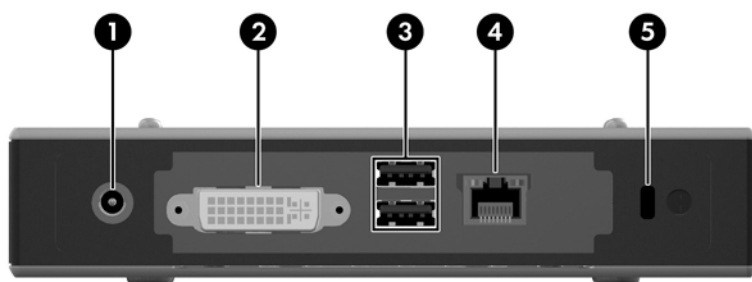
Afbeelding 3-1 Onderdelen op het achterpaneel
