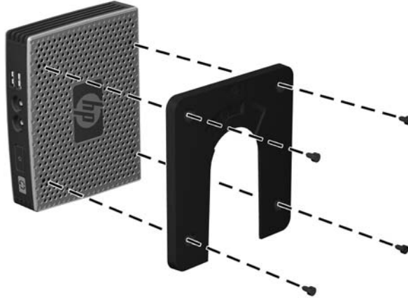
Afbeelding C-2 HP Quick Release aansluiten op de thin client
