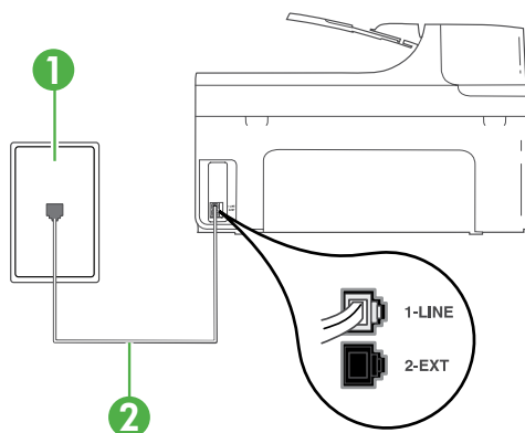
1 Zidna telefonska utičnica 2 Priključak 1-LINE na pislaču
