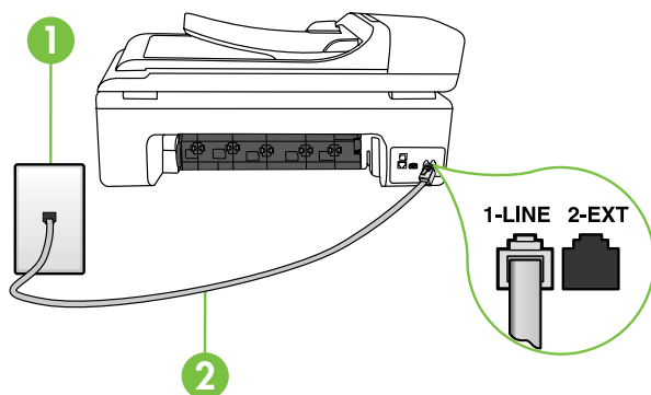
1 Prise téléphonique murale 2 Port 1-LINE de l'imprimante
