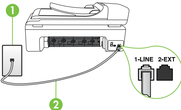
1: Telefónna zásuvka 2 Port 1-LINE na tlačiarňi
