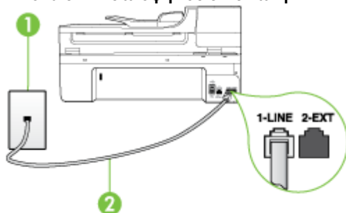
Εικόνα 8-1 Πίσω όψη του εκτυπωτή
