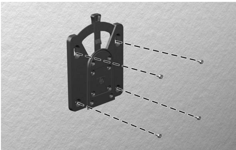
图 C-3 将 HP Quick Release 连接到另一设备
