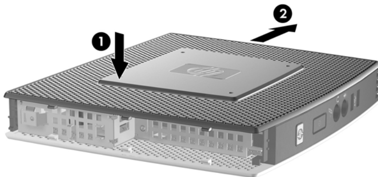
图 2-6 重新装上侧面检修面板
