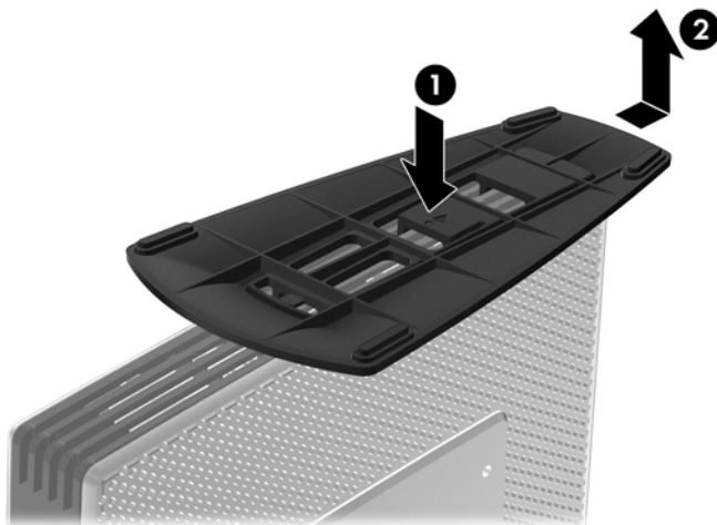
图 1-8 卸下底座
