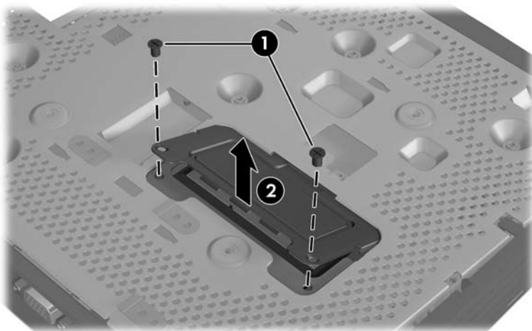
图 2-10 卸下 SO-DIMM 检修板
