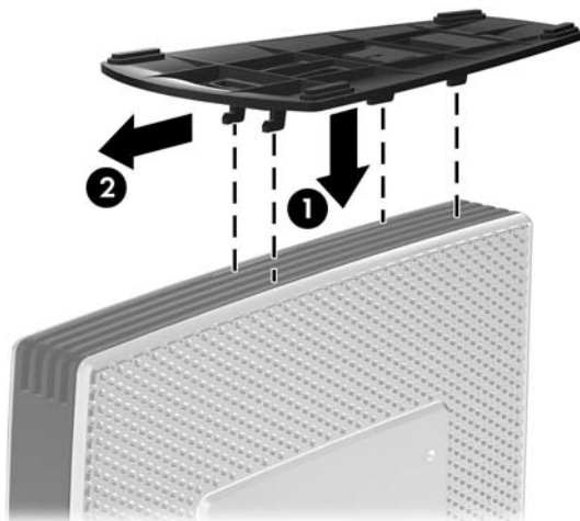
图 1-7 安装底座
