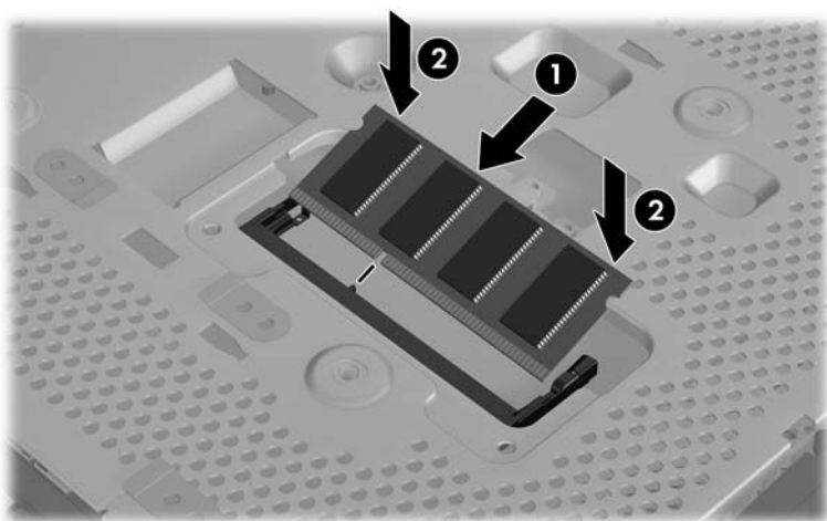
图 2-11 安装 SO-DIMM
