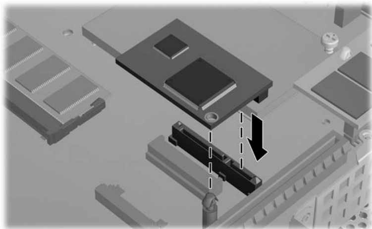
图 2-9 安装次要闪存模块
