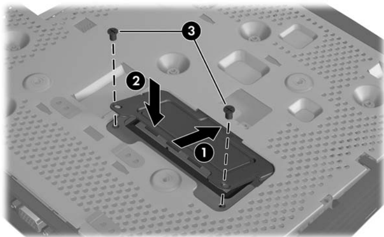
图 2-12 重新安装 SO-DIMM 检修板
