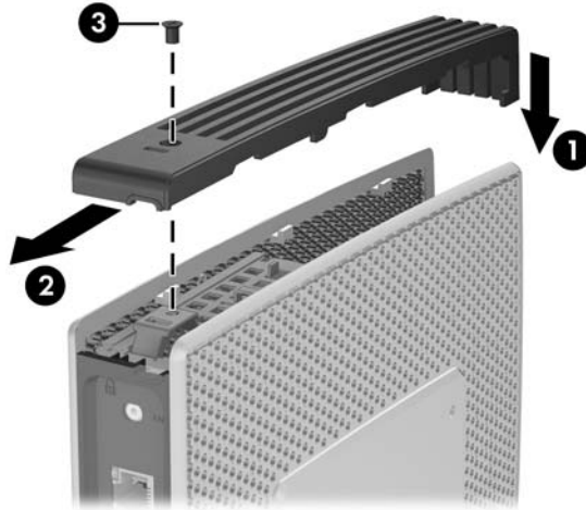
图 2-2 重新安装保护盒盖
