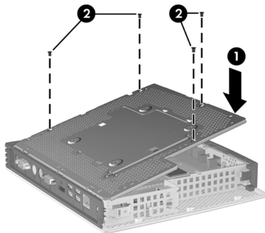
图 2-5 重新安装侧面金属盖
