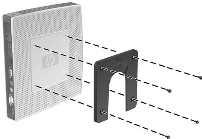
图 C-2 将 HP Quick Release 连接到瘦客户机
