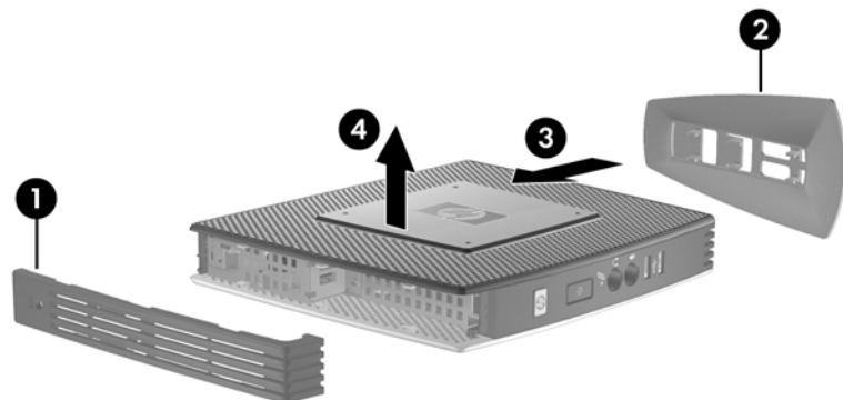
图 2-3 卸下侧面检修面板
