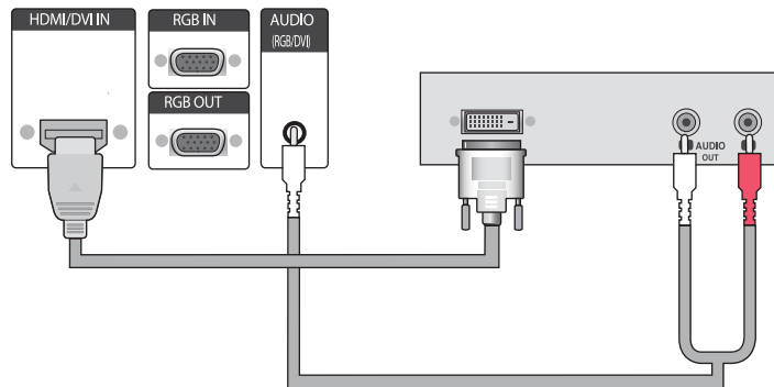
Figure 3-30 Connexion du câble de signal HDMI vers DVI
