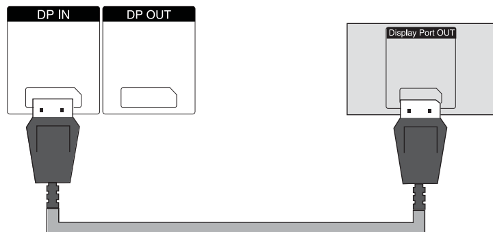
Figure 3-28 Connexion de l'entrée DisplayPort à un ordinateur ou lecteur multimédia
