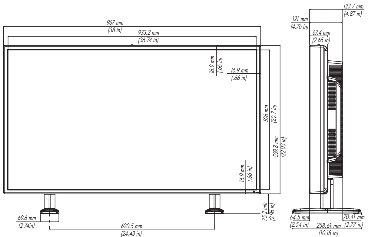
Figure B-1 HP LD4201 et HP LD4210 - Vues avant et latérale
