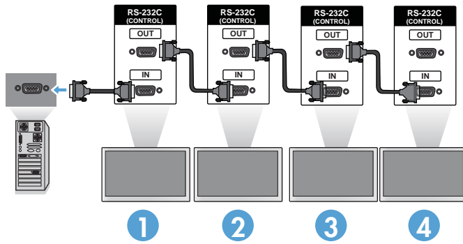
Figure 3-34 Connexion en cascade : RS-232-C
