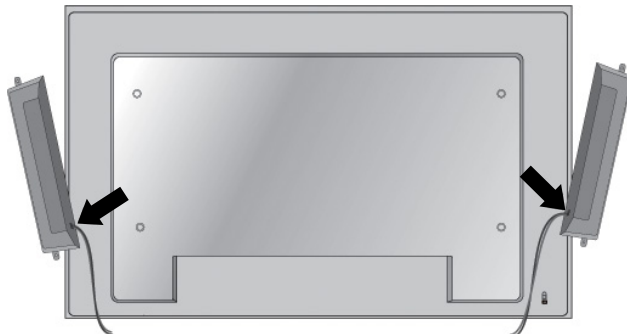
Figure 3-7 Montage des haut-parleurs
