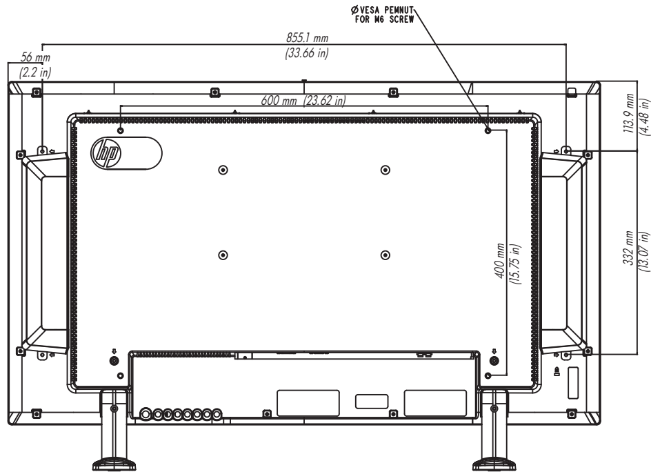
Figure B-2 HP LD4201 et HP LD4210 - Vue arrière
