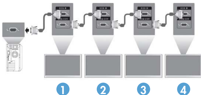
Figure 3-33 Connexion en cascade : RGB pour signal d'entrée vidéo
