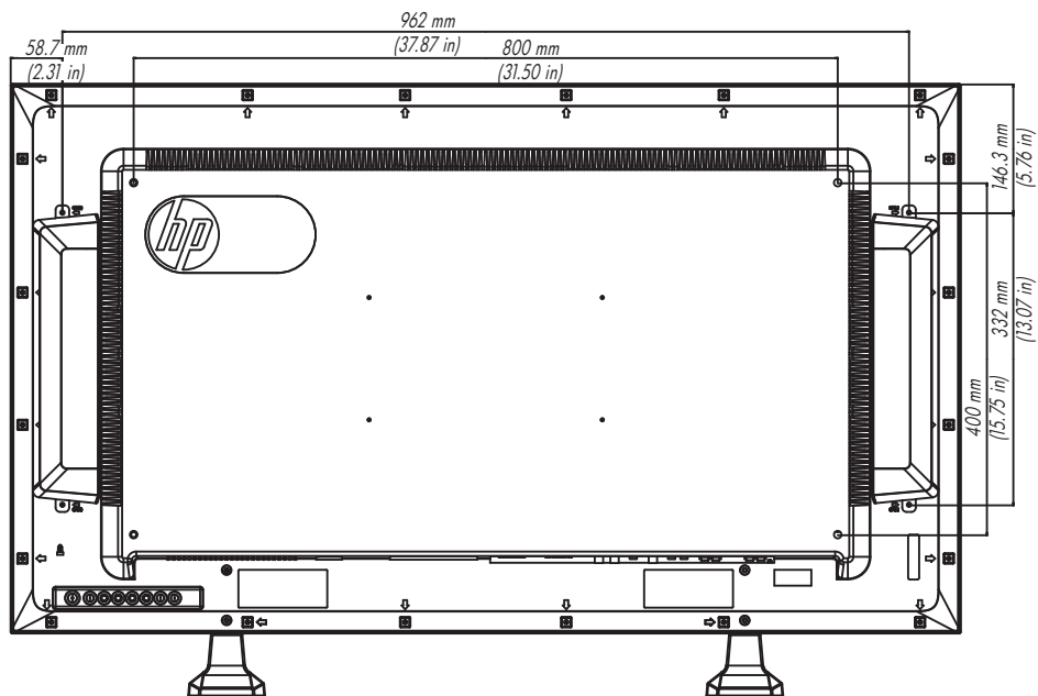
Figure B-4 HP LD4710 - Vue arrière
