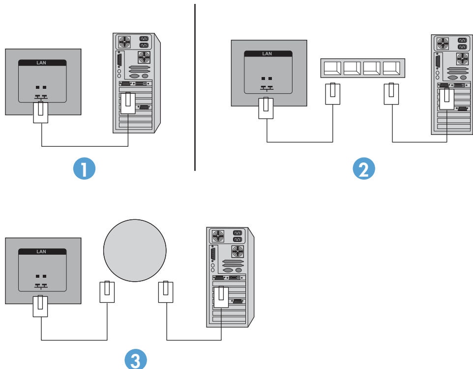
Figure 3-31 Connexion du câble réseau LAN
