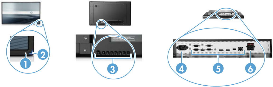
Figure 3-16 HP LD4710 - Composants de l'écran
