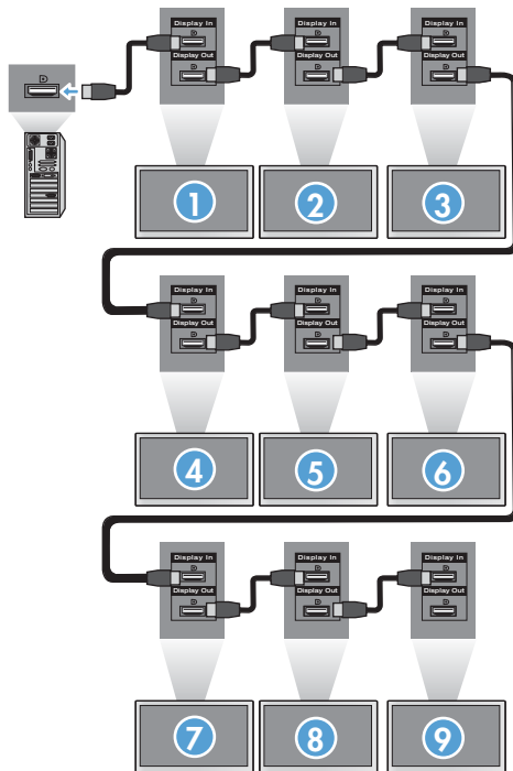
Figure 4-1 Mode mur d'image mur vidéo 3x3 : connexions d'écrans avec DP IN/DP OUT
