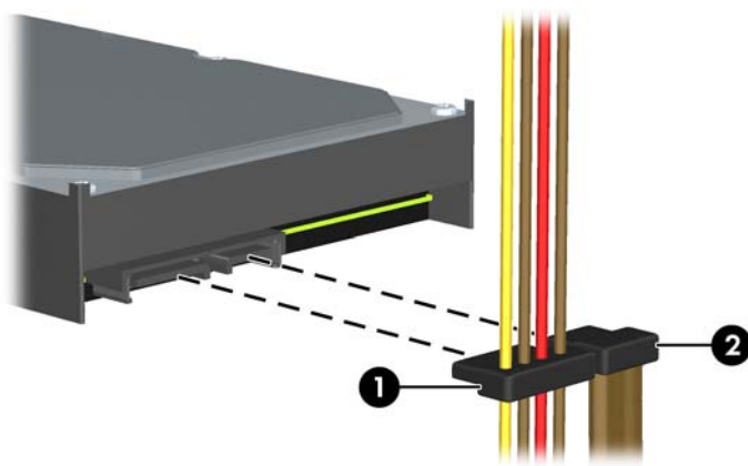
図 3-39 ハードディスク ドライブ ケーブルの接続
