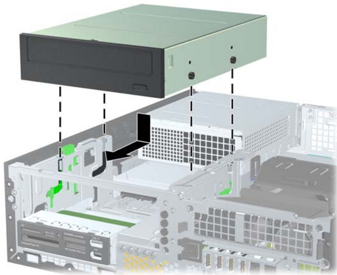
図 2-25 オプティカル ドライブの取り付け
