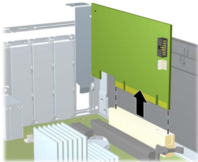
図 2-13 標準の PCI 拡張カードの取り外し
