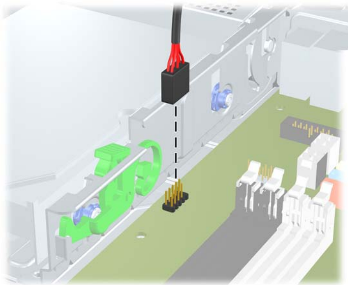
図 2-30 メディア カード リーダーの 1394 ケーブルの取り外し
