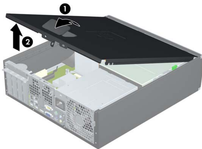
図 2-1 アクセス パネルの取り外し
