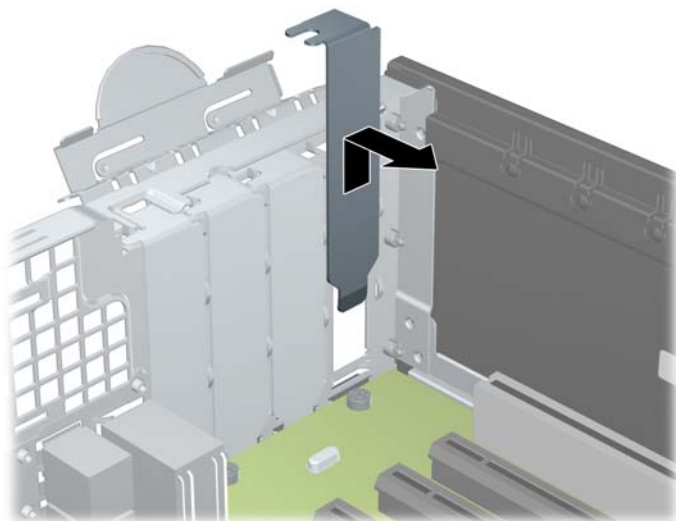
図 3-11 拡張スロット カバーの取り外し
