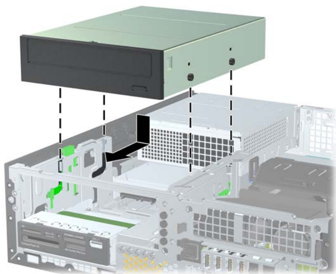
図 3-23 オプティカル ドライブの取り付け
