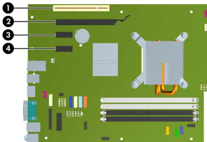
図 2-10 拡張スロットの位置
