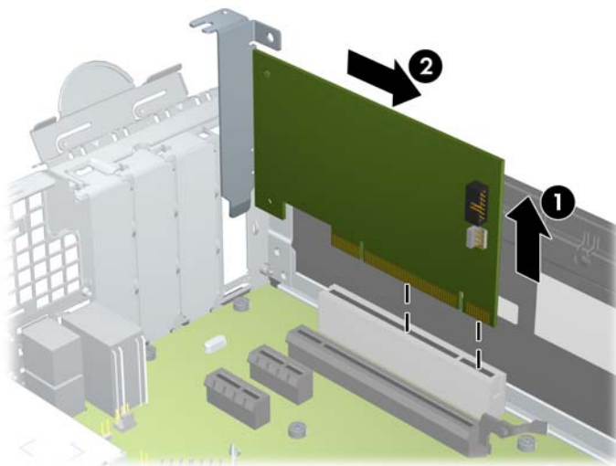
图 3-12 卸下标准 PCI 扩展卡
