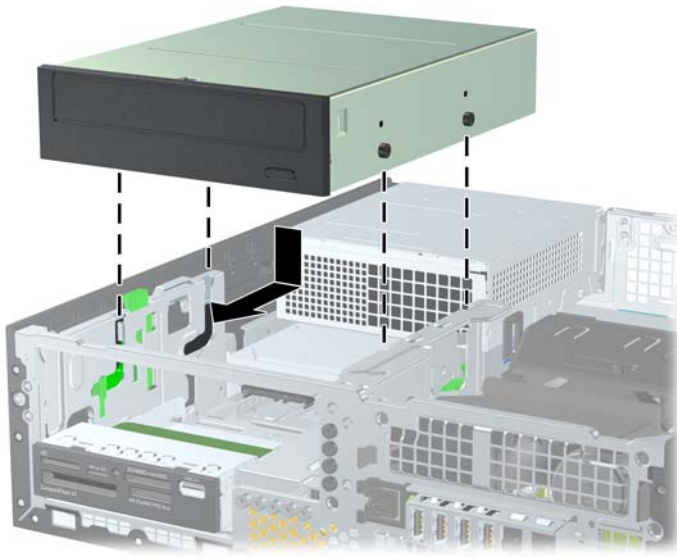
图 3-23 安装光驱
