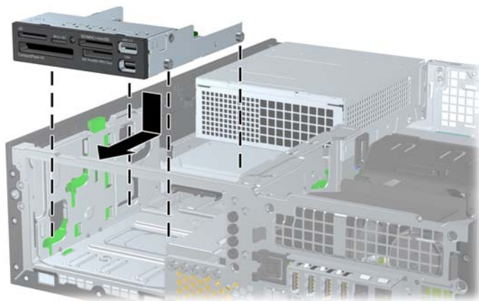
图 2-32 将驱动器安装到 3.5 英寸驱动器安托架中（所示为介质卡读卡器）
