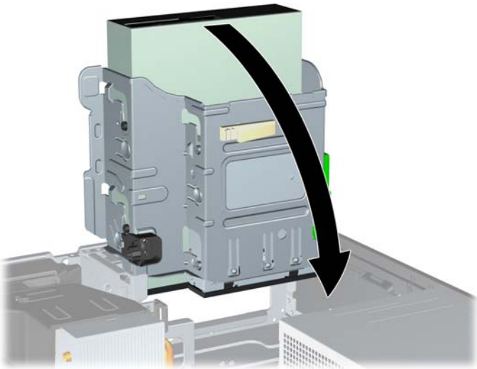
图 3-20 向下转动驱动器框架
