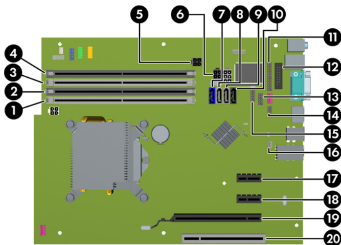
图 3-7 主板连接
