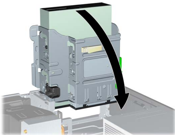
图 2-22 向下转动驱动器框架
