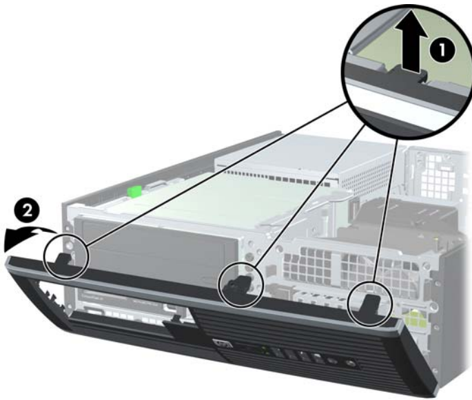
图 2-3 卸下前面板
