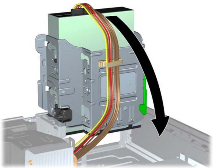
图 3-26 向下转动驱动器框架
