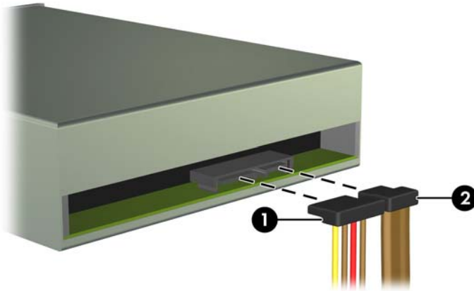
图 3-19 断开电源电缆和数据电缆
