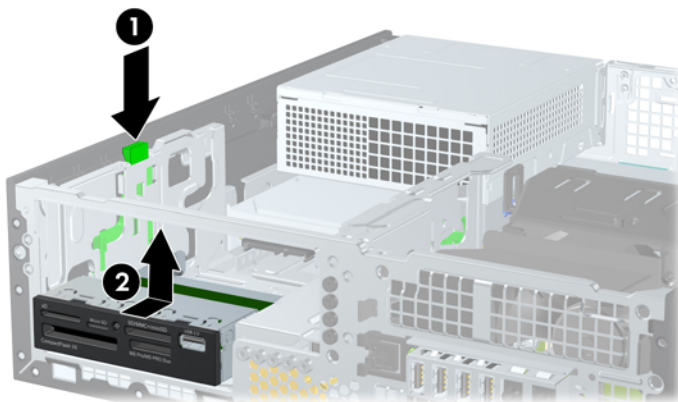
图 3-28 卸下 3.5 英寸驱动器（所示为介质卡读卡器）
