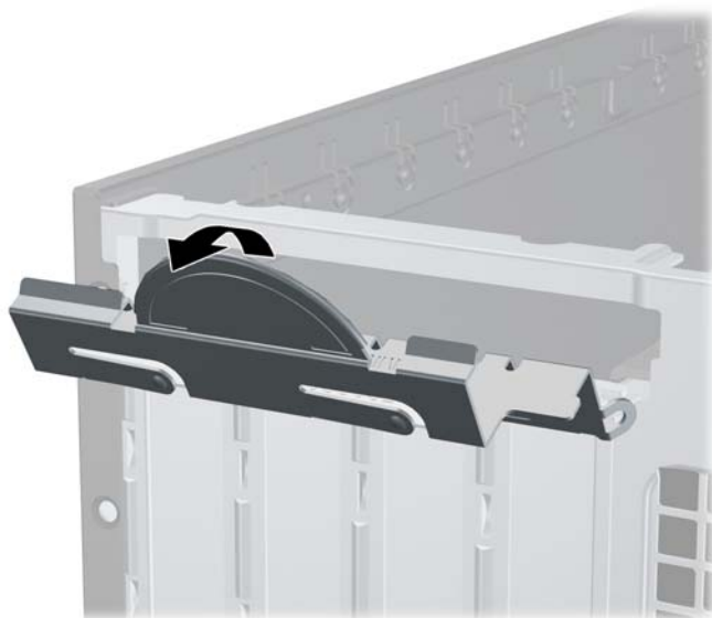
图 2-11 打开扩展槽固定器
