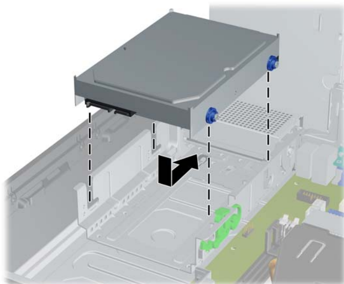
图 2-38 安装硬盘驱动器
