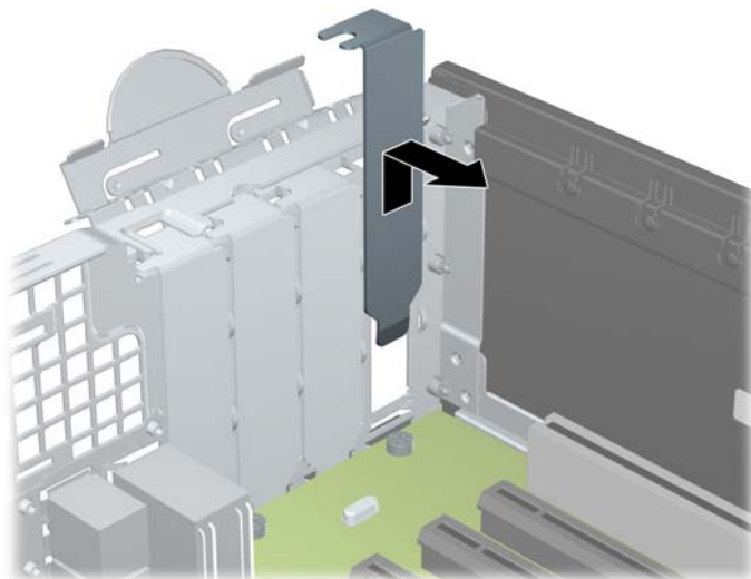
图 3-11 卸下扩展槽挡片
