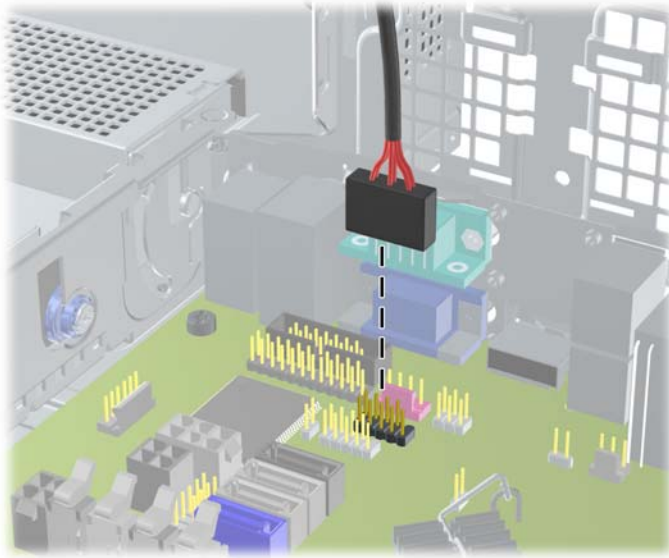
图 3-27 断开介质卡读卡器 USB 电缆
