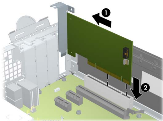
图 3-14 安装扩展卡
