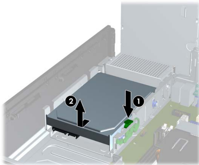
图 2-36 卸下硬盘驱动器
