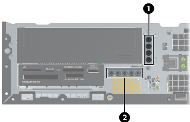
图 3-17 额外导向螺钉的位置
