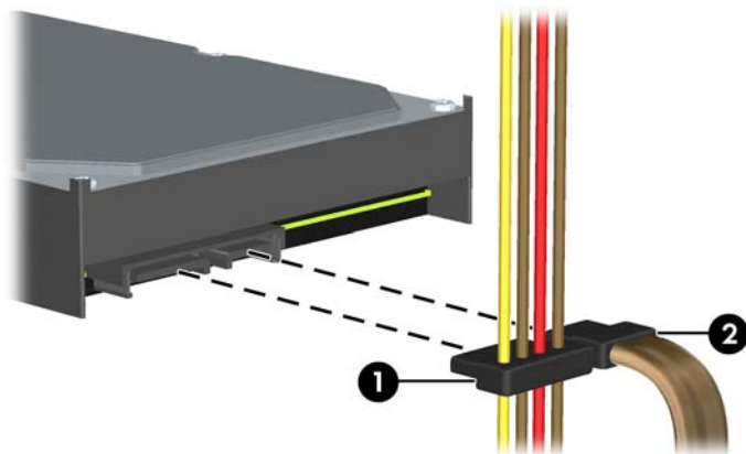
图 3-31 连接辅助硬盘驱动器电源电缆和数据电缆
