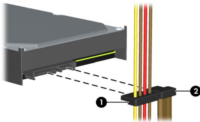
图 3-39 连接硬盘驱动器电缆
