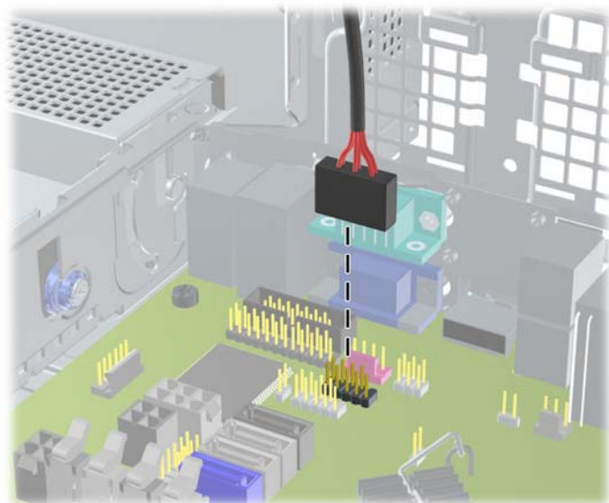
图 3-32 连接介质卡读卡器 USB 电缆
