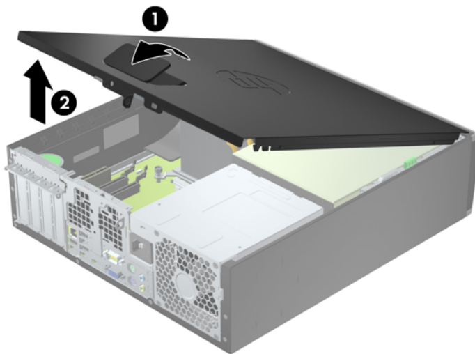
图 3-1 卸下计算机检修面板
