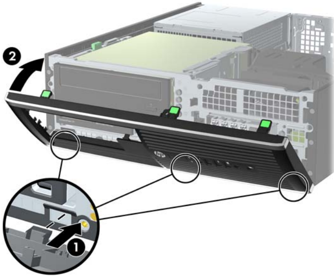
图 3-5 重新装上前面板
