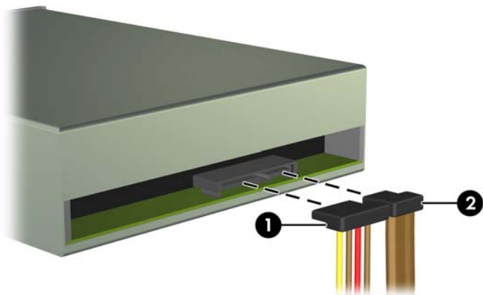
图 3-25 连接电源线和数据电缆
