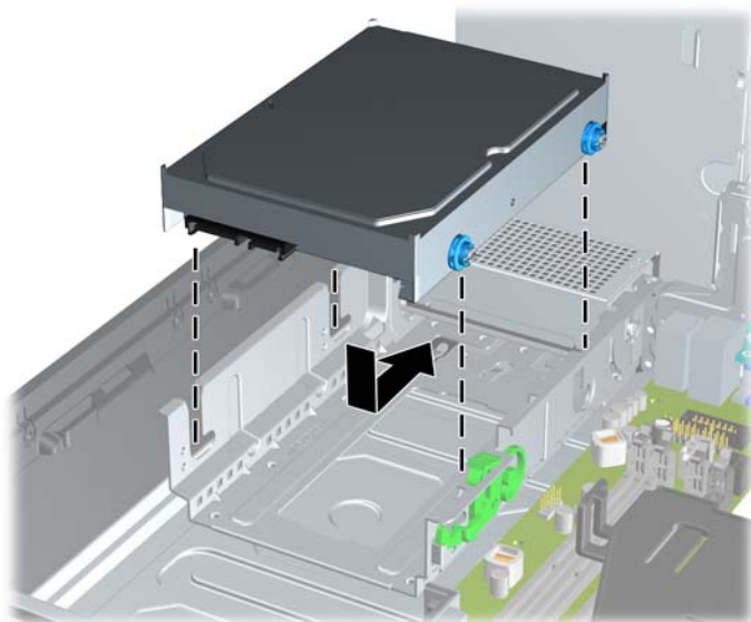
图 3-38 安装硬盘驱动器
