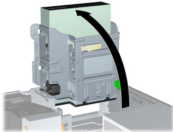
图 3-24 向上转动驱动器框架
