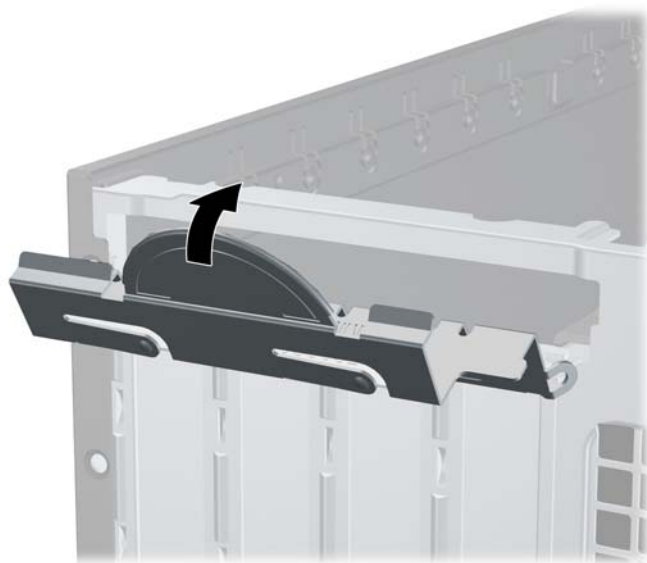
图 3-15 关闭扩展槽固定器
