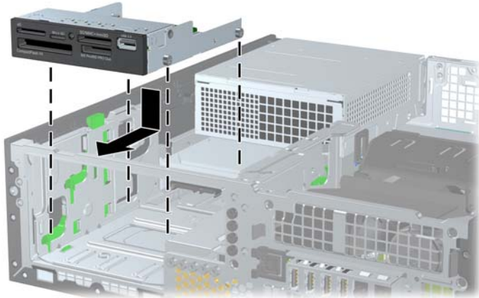
图 3-30 将驱动器安装到 3.5 英寸驱动器安托架中（所示为介质卡读卡器）
