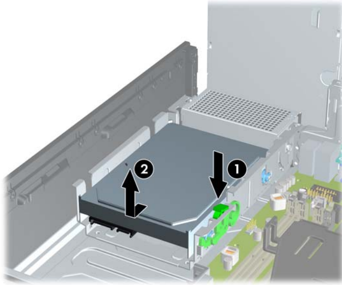
图 3-36 卸下硬盘驱动器
