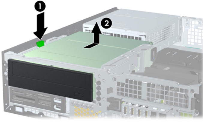
图 2-23 卸下 5.25 英寸驱动器
