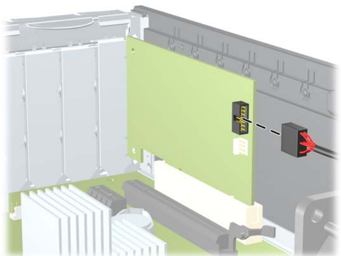
图 2-30 断开介质卡读卡器 1394 电缆
