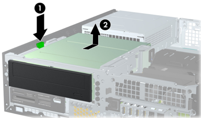
图 3-21 卸下 5.25 英寸驱动器
