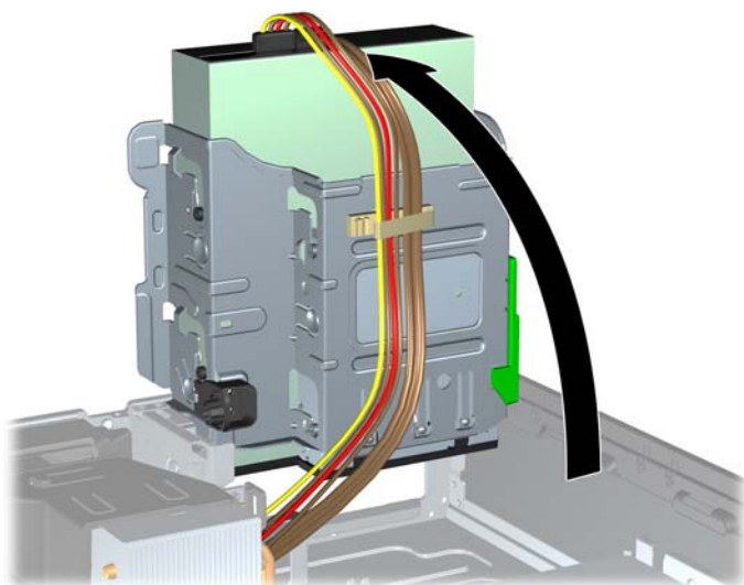
图 3-33 向上转动驱动器框架
