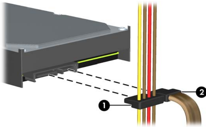
图 3-35 断开硬盘驱动器电缆
