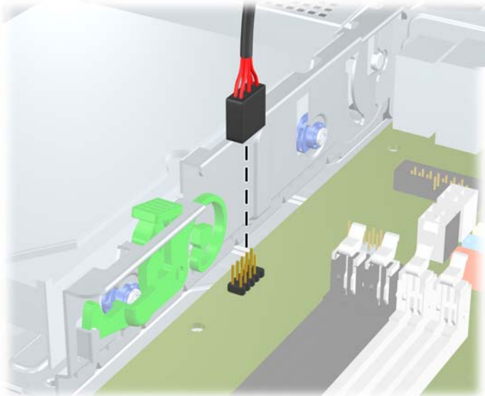
圖示 2-30 拔除讀卡機 1394 纜線
