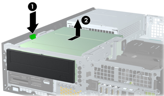
圖示 3-21 拆下 5.25 英寸磁碟機
