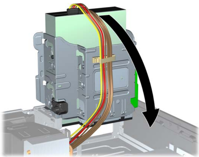
圖示 3-26 將磁碟機裝架向下翻轉
