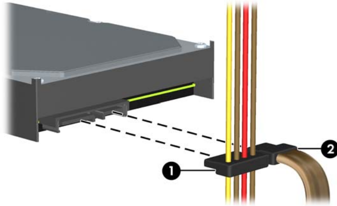
圖示 3-31 連接第二硬碟機電源線和資料排線
