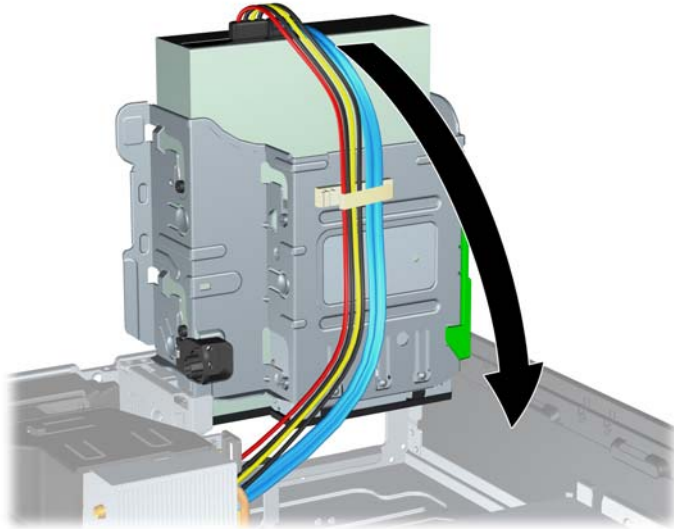
圖示 2-28 將磁碟機裝架向下翻轉
