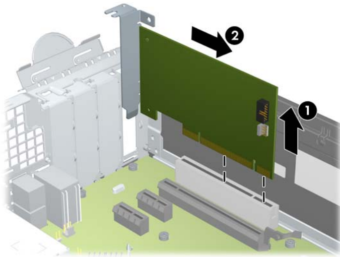
圖示 3-12 拆下標準 PCI 擴充卡
