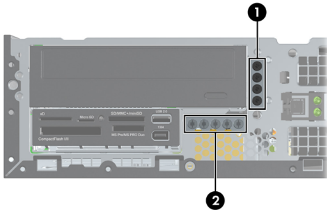
圖示 2-18 額外的導引螺絲位置
