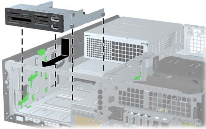
圖示 2-32 將磁碟機安裝至 3.5 英吋磁碟機插槽（所示為讀卡機）
