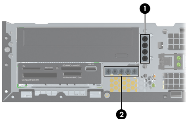
圖示 3-17 額外的導引螺絲位置
