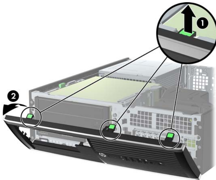
圖示 3-3 移除前面板
