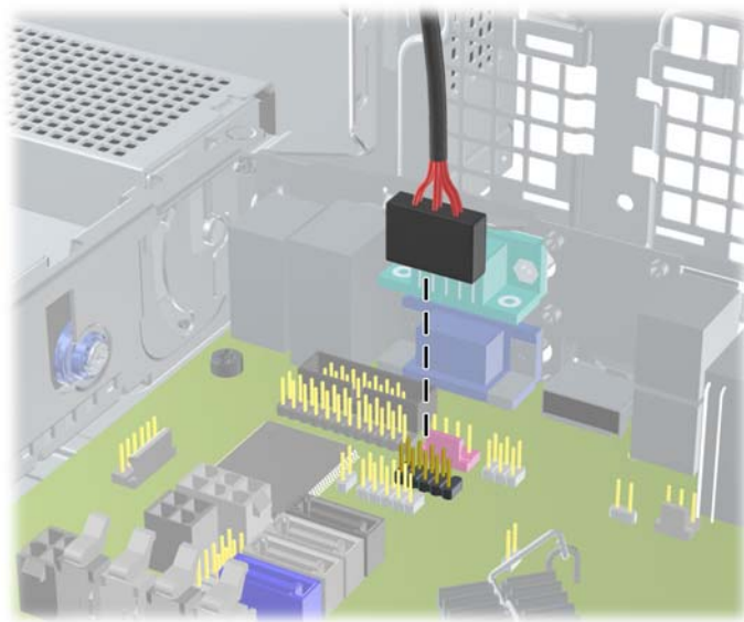
圖示 3-32 連接讀卡機的 USB 纜線
