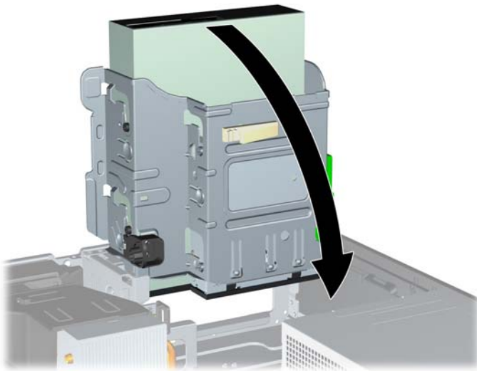
圖示 2-22 將磁碟機裝架向下翻轉
