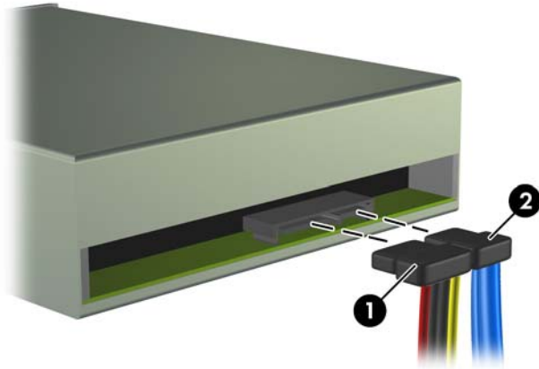
圖示 2-21 拔除電源線和資料排線
