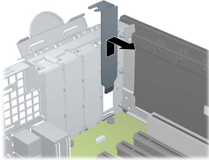
圖示 3-11 拆下擴充槽擋板
