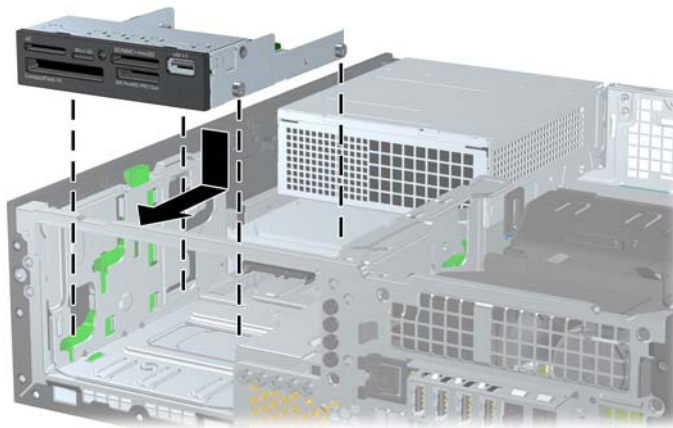
圖示 3-30 將磁碟機安裝至 3.5 英寸磁碟機插槽（所示為讀卡機）
