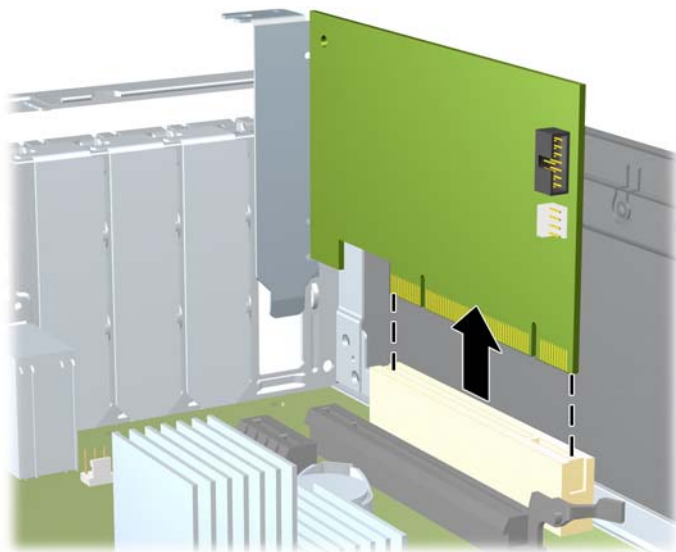
圖示 2-13 拆下標準 PCI 擴充卡
