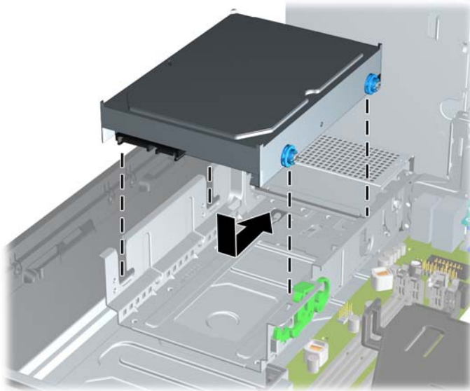
圖示 3-38 安裝硬碟機
