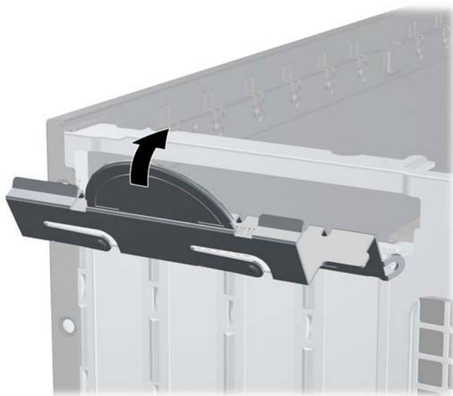
圖示 3-15 關閉擴充槽固定器
