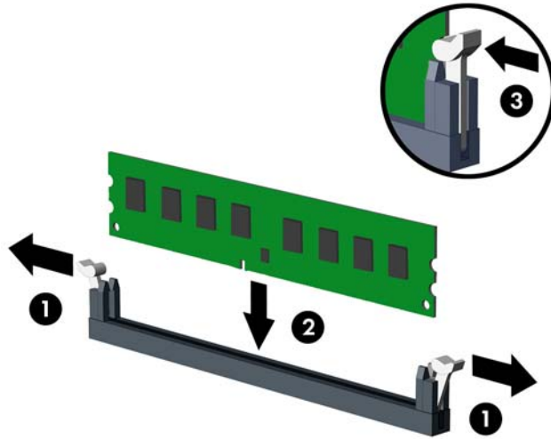
圖示 2-9 安裝 DIMM
