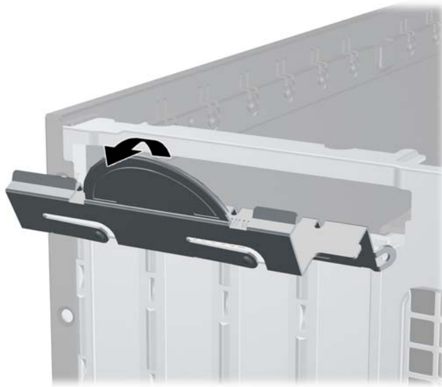
圖示 2-11 打開擴充槽支架
