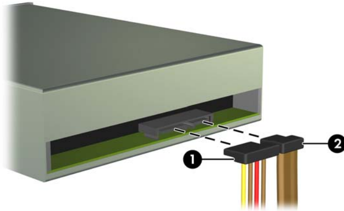
圖示 3-19 拔除電源線和資料排線
