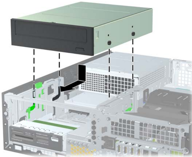
圖示 3-23 安裝光碟機
