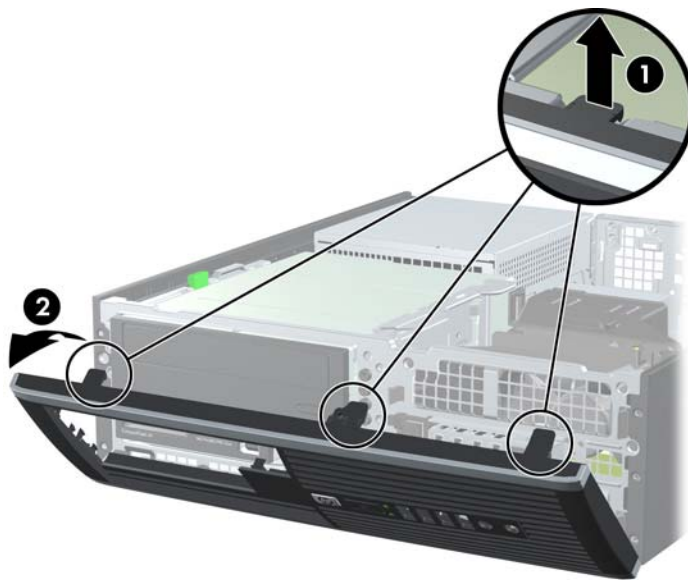
圖示 2-3 拆下前面板
