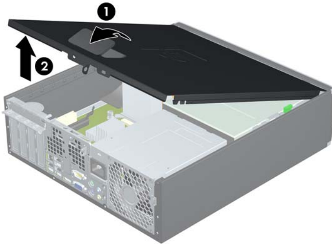
圖示 2-1 拆下存取面板
