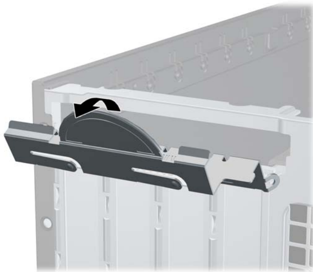
圖示 3-10 打開擴充槽支架
