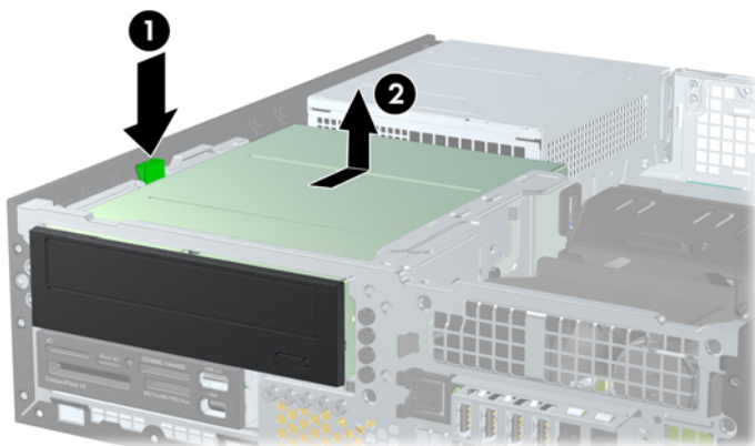
圖示 2-23 拆下 5.25 英吋磁碟機
