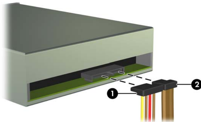
圖示 3-25 連接電源線和資料排線
