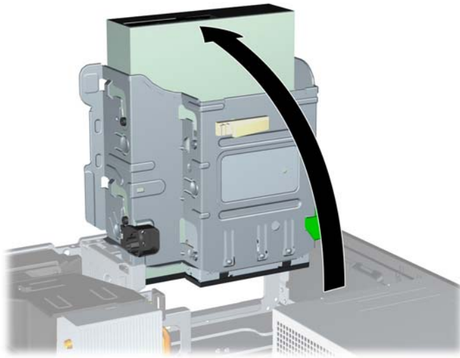
圖示 2-26 將磁碟機裝架向上翻轉
