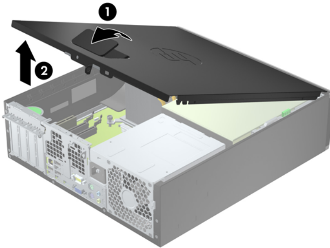
圖示 3-1 拆下電腦存取面板
