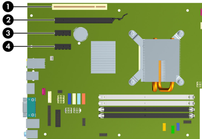
圖示 2-10 擴充槽位置
