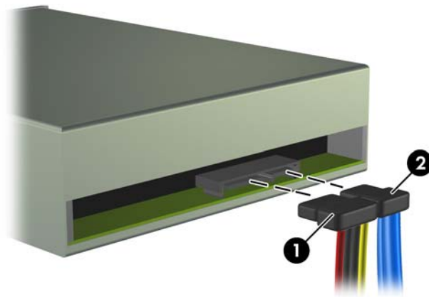
圖示 2-27 連接電源線和資料排線
