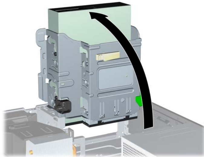
圖示 3-24 將磁碟機裝架向上翻轉
