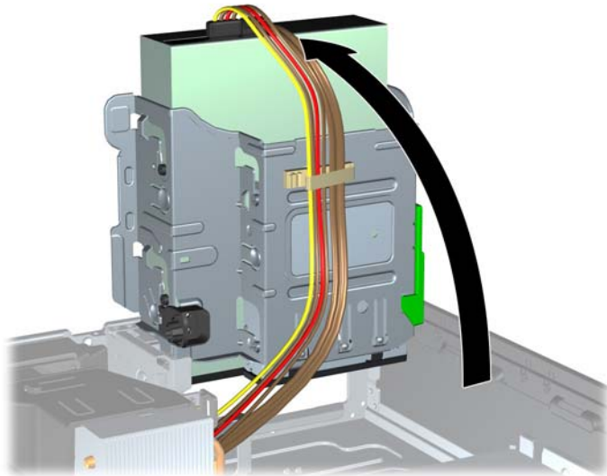
圖示 3-18 將磁碟機裝架向上翻轉
