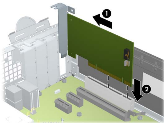
圖示 3-14 安裝擴充卡
