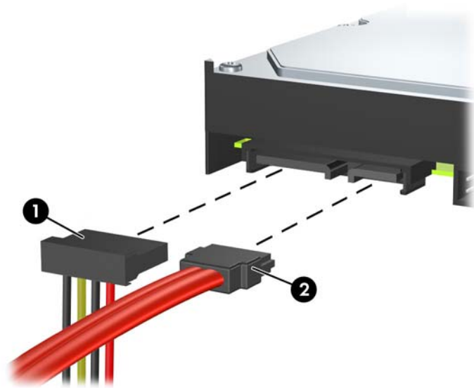
圖示 2-35 拔除硬碟機電源線和資料排線
