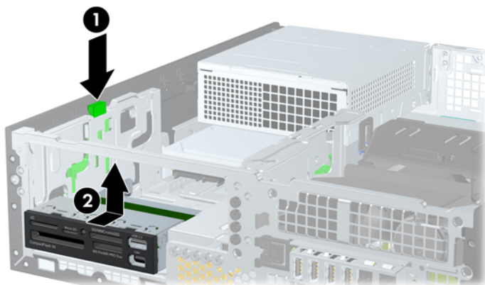
圖示 2-31 拆下 3.5 英吋磁碟機 (所示為讀卡機)
