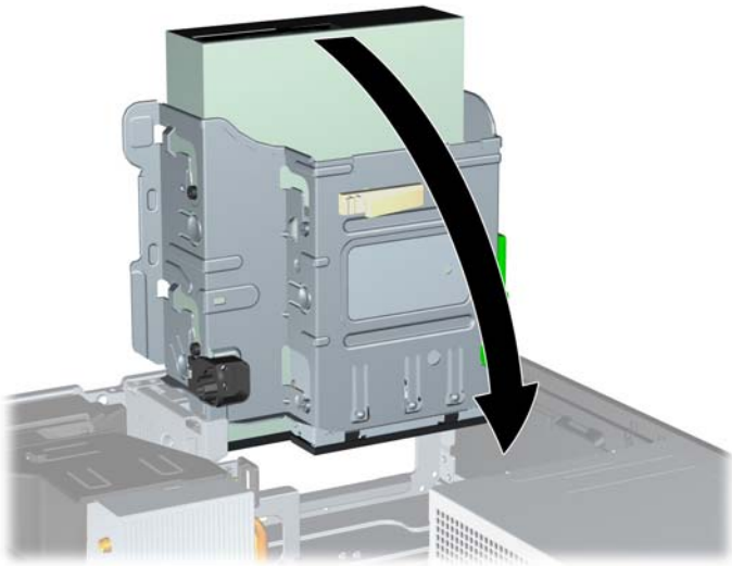
圖示 3-20 將磁碟機裝架向下翻轉
