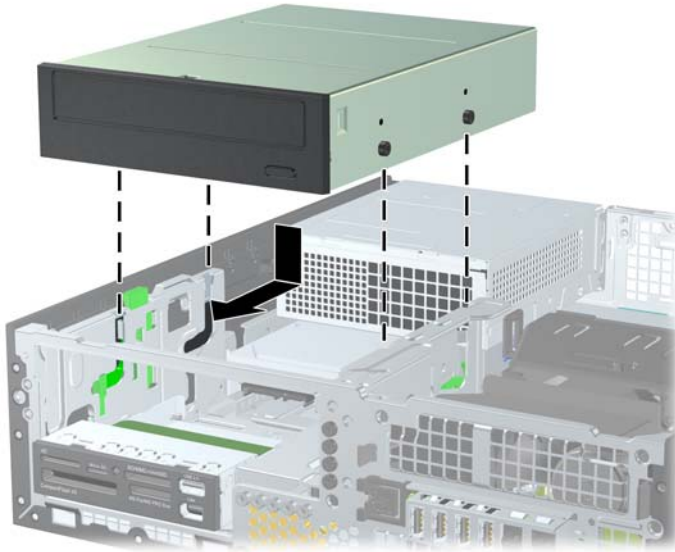
圖示 2-25 安裝光碟機
