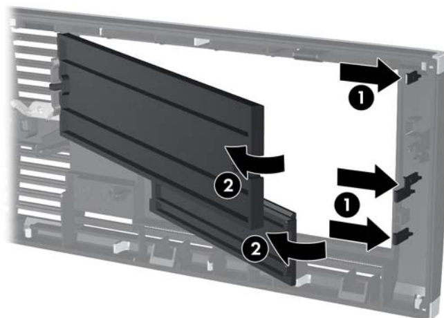
圖示 3-4 拆下機殼擋板
