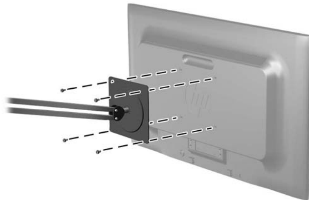
Figura 3-8 Installazione del monitor
