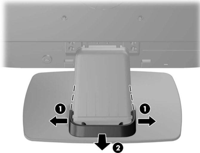
Figura 3-3 Rimozione del braccio di supporto cavi
