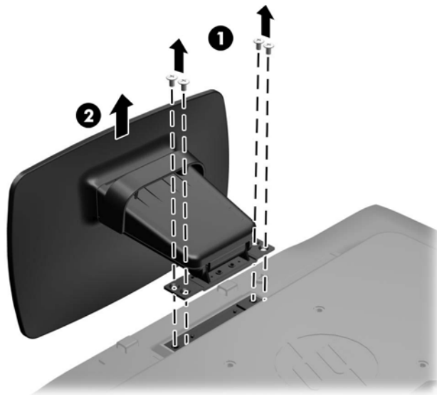
Figura 3-7 Rimozione delle viti dal piedistallo
