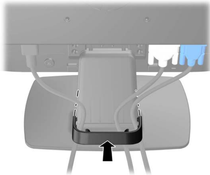
Figura 3-5 Installazione del braccio di supporto per i cavi
