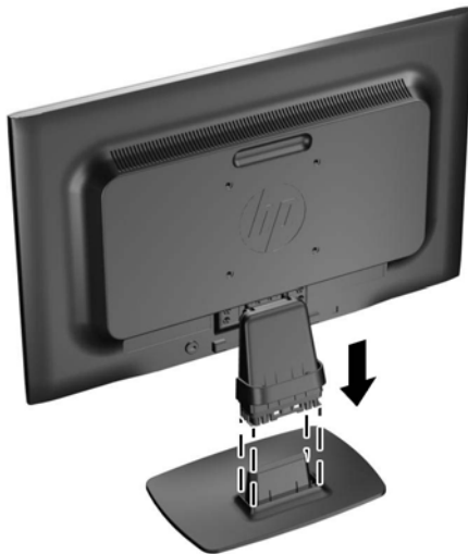
Figura 3-1 Montaggio della base del monitor
