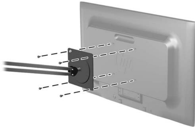
그림 3-8 모니터 장착
