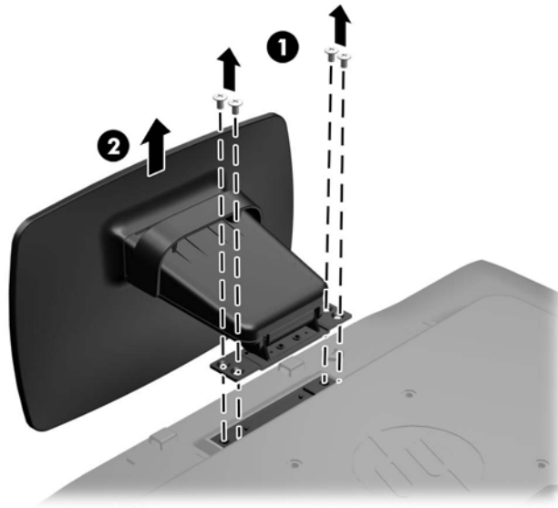
그림 3-7 모니터 받침대 목 나사 제거
