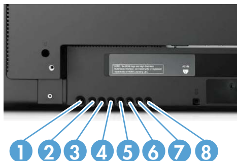
Εικόνα 3-18 HP LD4720tm—Πίνακας ελέγχου οθόνης
