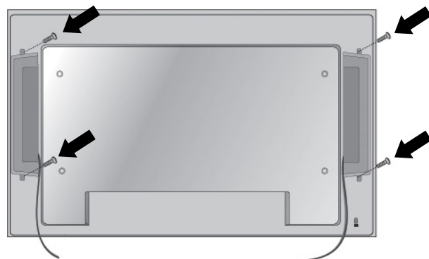
Εικόνα 3-8 Στερέωση των ηχείων στην οθόνη
