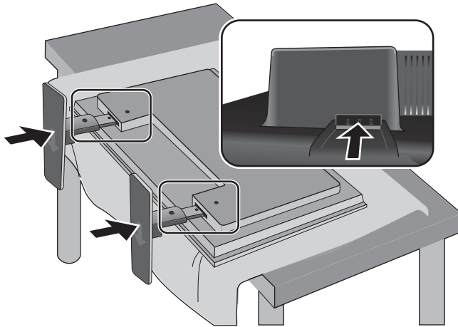
Εικόνα 3-4 HP LD4720tm—Ολίσθηση της βάσης πάνω στην οθόνη
