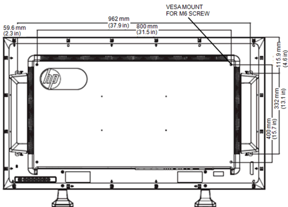
Εικόνα B-4 HP LD4720tm—Πίσω όψη
