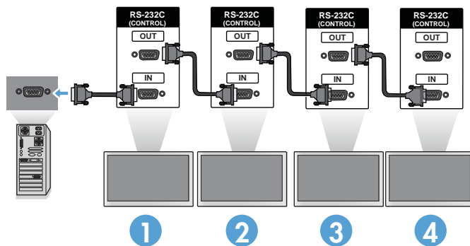
Εικόνα 3-35 Αλυσιδωτή σύνδεση—RS-232-C
