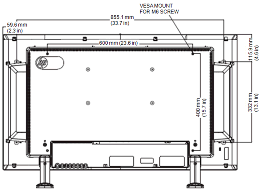
Εικόνα B-2 HP LD4220tm—Πίσω όψη
