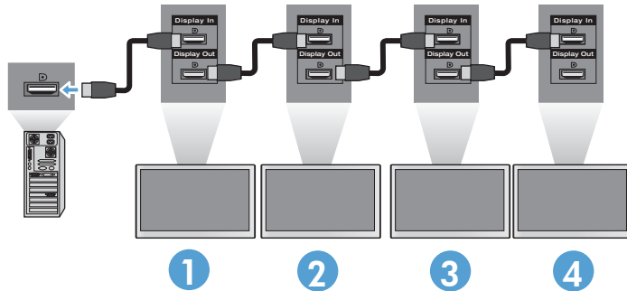
Εικόνα 3-34 Αλυσιδωτή σύνδεση—RGB για σήμα εισόδου βίντεο
