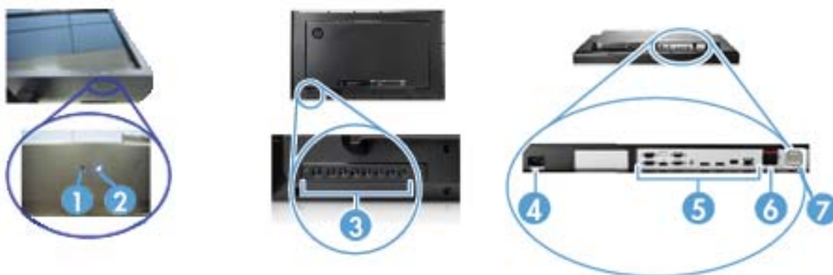
Εικόνα 3-16 HP LD4720tm—Εξαρτήματα οθόνης
