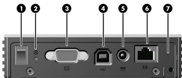
図 2-1 リア パネルの各部
