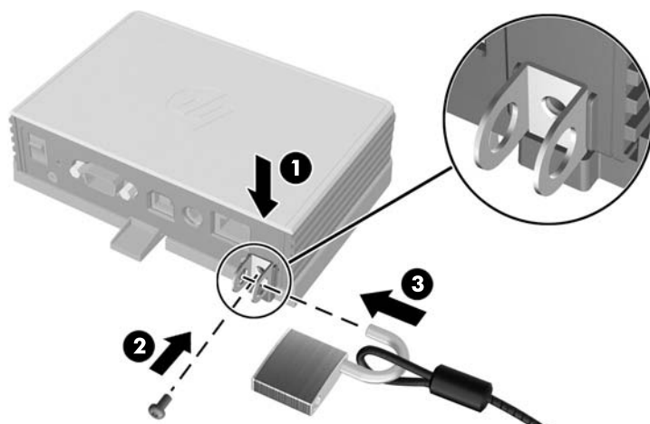
図 B-2 設置ブラケットへの t200 Zero Client の固定
