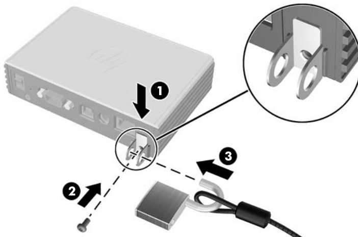
図 B-1 t200 Zero Client の固定
