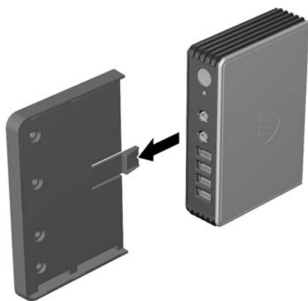
図 C-1 設置ブラケットへの t200 Zero Client の挿入
