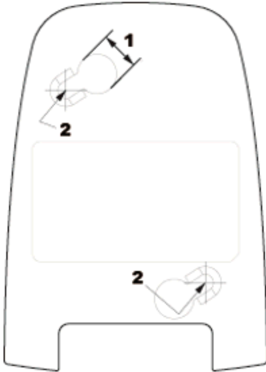
Εικόνα 1-1 Πατρών οπών βιδών
