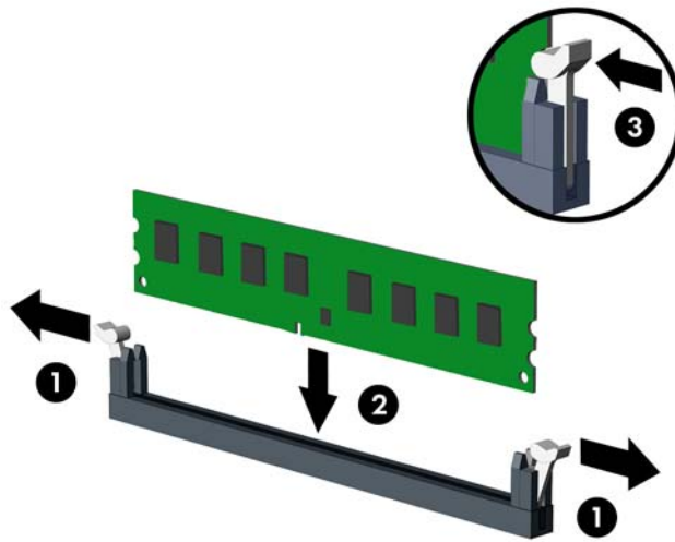
Figura 2-7 Instalación de DIMM
