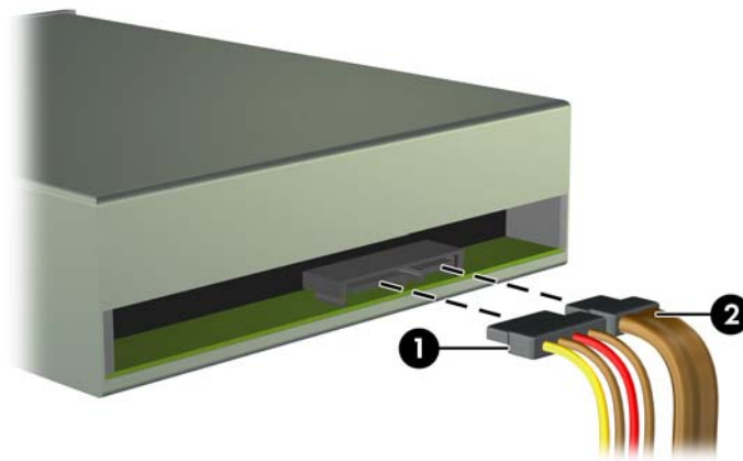
Figura 3-17 Desconexión de los cables de la unidad óptica
