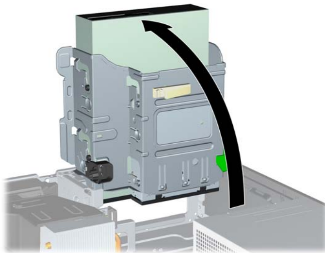
Figura 4-24 Giro del compartimiento para unidades a la posición vertical
