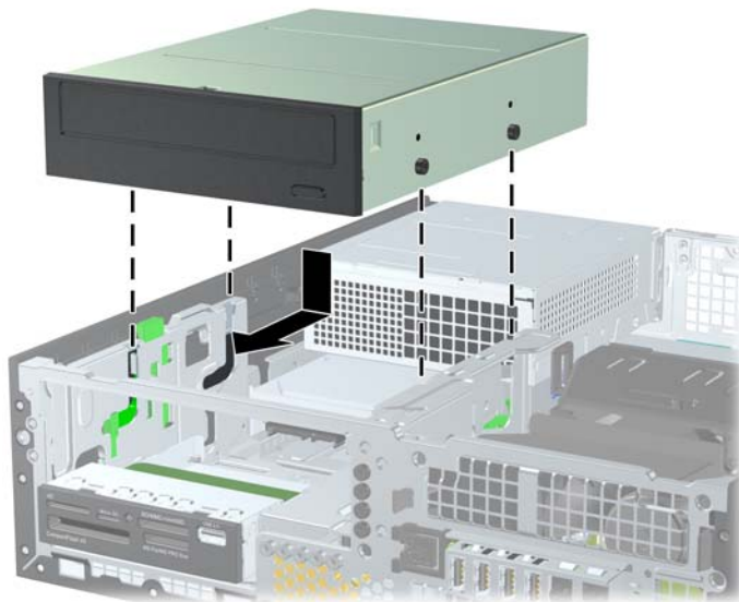
Figura 4-23 Instalación de la unidad óptica
