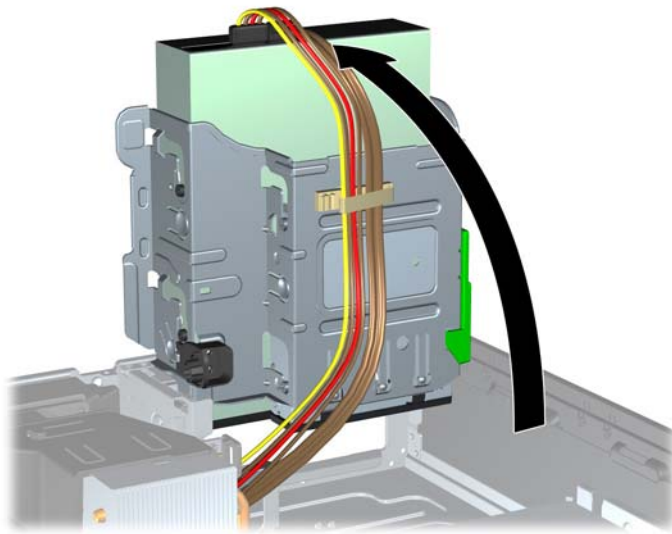
Figura 4-33 Giro del compartimiento para unidades a la posición vertical
