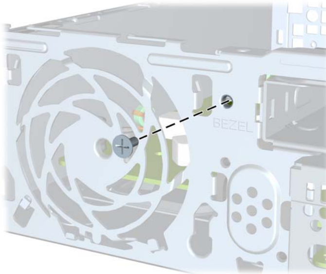
Figura 5-35 Extracción del tornillo de seguridad del panel frontal
