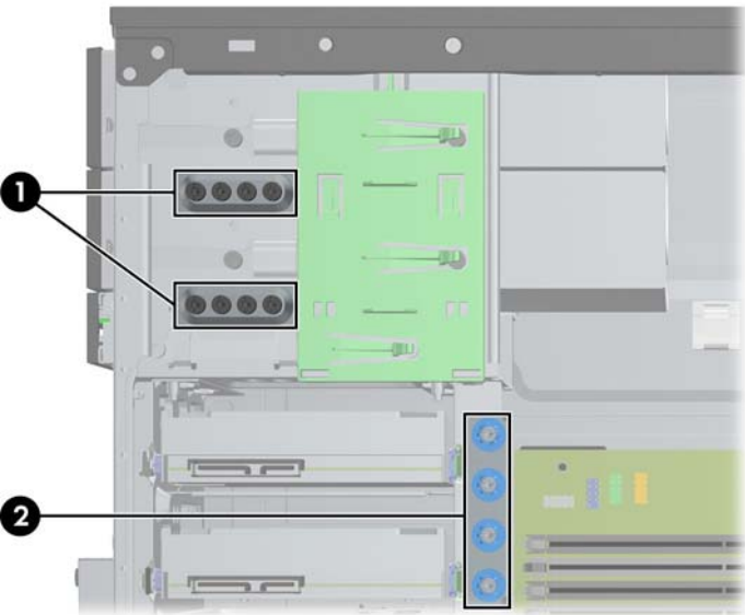
Figura 3-16 Ubicación de los tornillos guía adicionales
