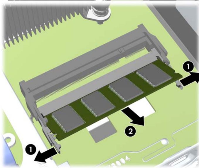
Figura 5-10 Extracción de un SODIMM
