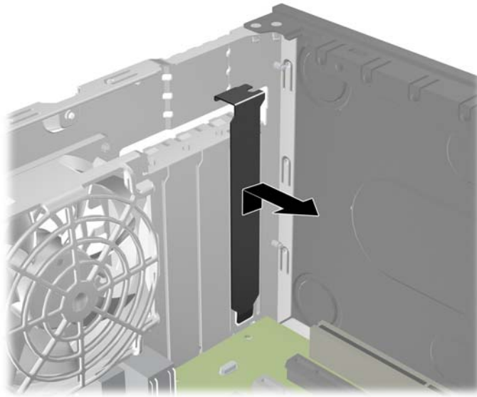
Figura 3-10 Extracción de la cubierta de la ranura de expansión
