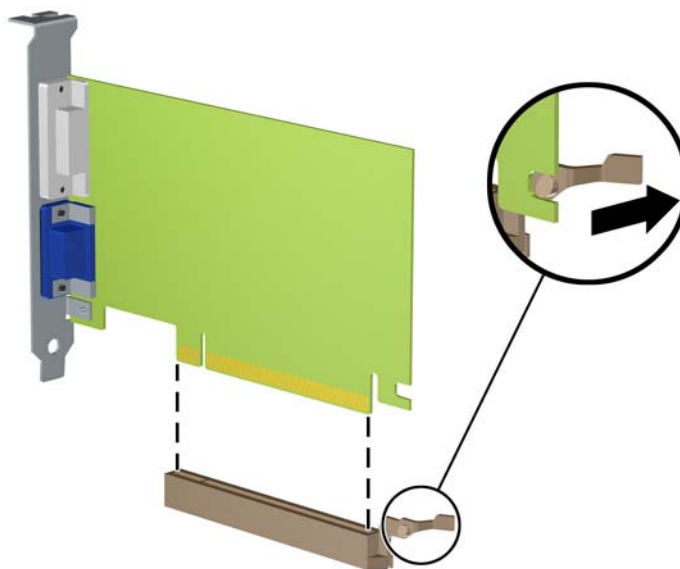
Figura 3-12 Extracción de una tarjeta de expansión PCI Express x16
