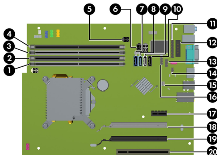
Figura 4-7 Conexiones de la placa del sistema
