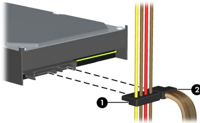
Figura 4-31 Conexión de los cables de alimentación y de datos de la unidad de disco duro secundaria
