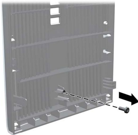
Figura 3-42 Extracción del tornillo de seguridad del panel frontal
