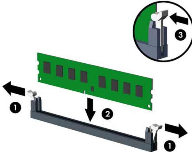
Figura 4-9 Instalación de DIMM
