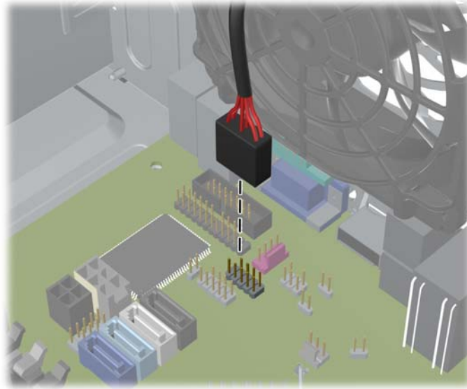
Figura 3-23 Conexión del cable USB del lector de tarjetas multimedia
