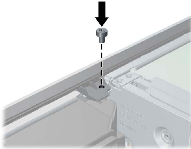
Figura 4-51 Instalación del tornillo de seguridad en el panel frontal
