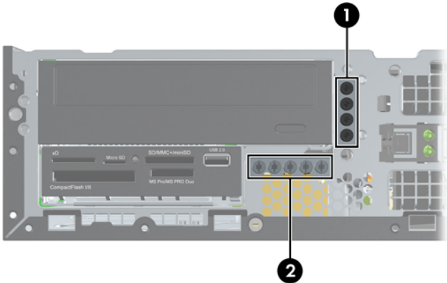
Figura 4-17 Ubicación de los tornillos guía adicionales
