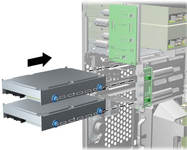
Figura 3-30 Introducción de una unidad de disco duro en el compartimiento para unidades
