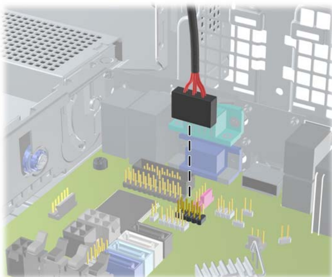
Figura 4-27 Desconexión del cable USB del lector de tarjetas multimedia
