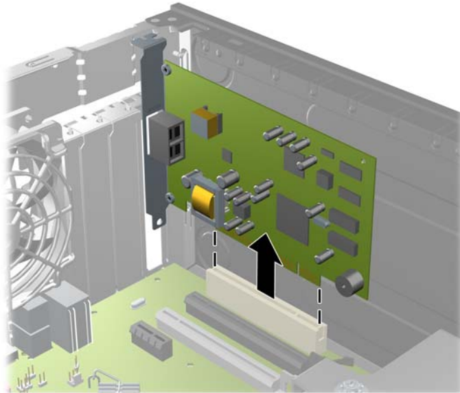
Figura 3-11 Extracción de la tarjeta de expansión PCI estándar
