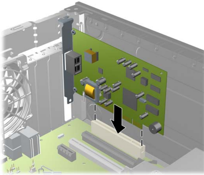
Figura 3-13 Instalación de una tarjeta de expansión
