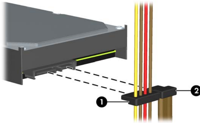
Figura 3-24 Desconexión de los cables de la unidad de disco duro
