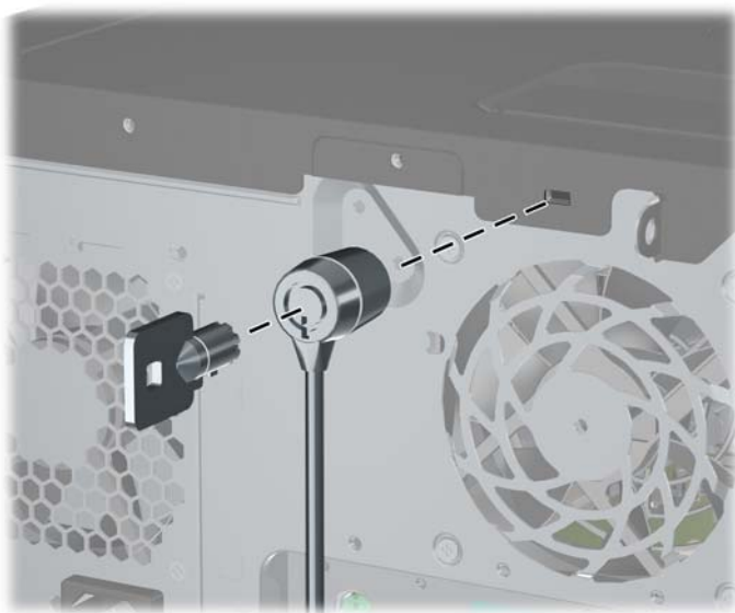
Figura 2-39 Instalación de un bloqueo de cable
