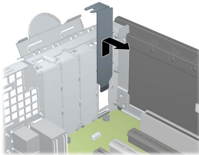
Figura 4-11 Extracción de la cubierta de la ranura de expansión
