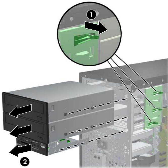
Figura 3-19 Extracción de unidades
