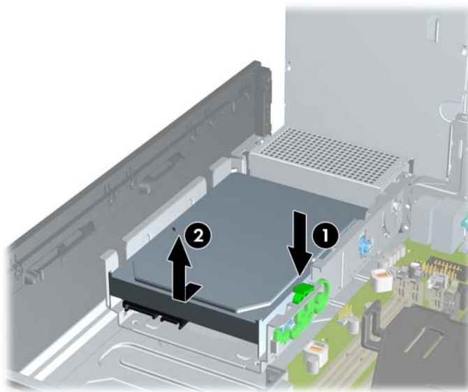
Figura 4-36 Extracción de la unidad de disco duro
