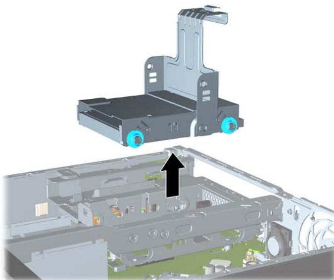
Figura 5-16 Extracción del transportador de la unidad de disco duro
