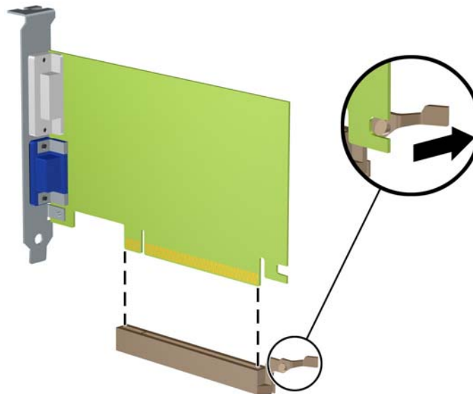
Figura 4-13 Extracción de una tarjeta de expansión PCI Express x16
