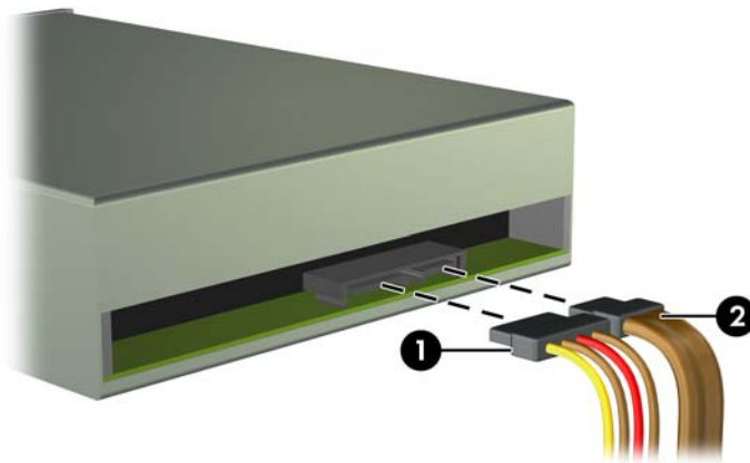
Figura 3-22 Conexión de los cables de la unidad óptica
