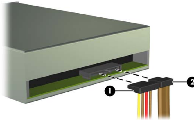
Figura 4-19 Desconexión de los cables de alimentación y de datos
