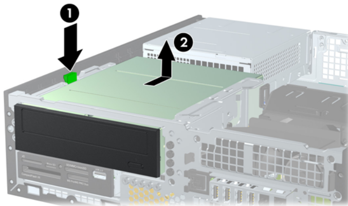
Figura 4-21 Extracción de una unidad de 5,25 pulgadas
