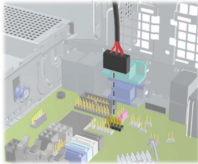
Figura 4-32 Conexión del cable USB del lector de tarjetas multimedia
