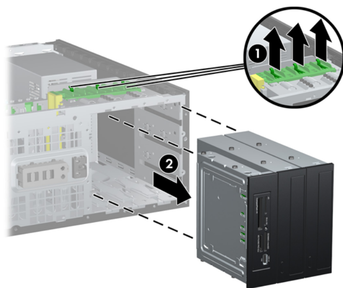
Figura 2-33 Liberación de las unidades de 5,25 pulgadas de los compartimientos (Minitorre)
