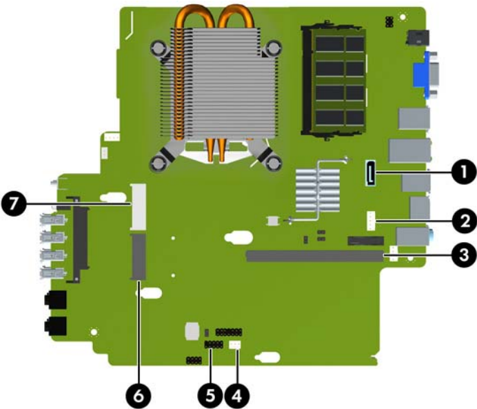
Figura 5-8 Conexiones de la placa del sistema
