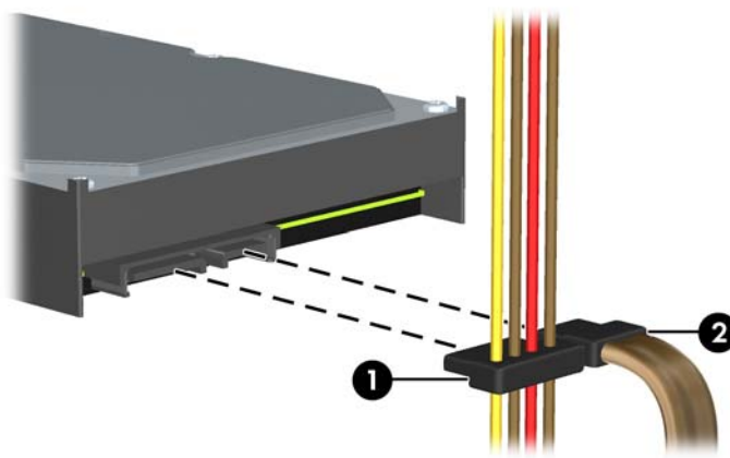
Figura 4-35 Desconexión de los cables de la unidad de disco duro
