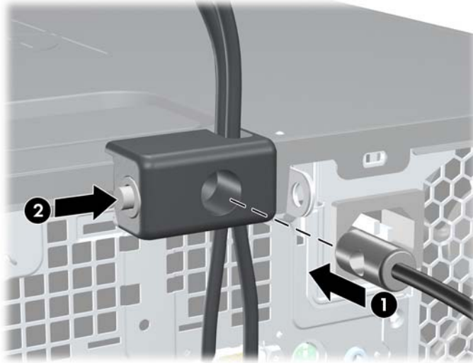
Figura 4-48 Activación del bloqueo
