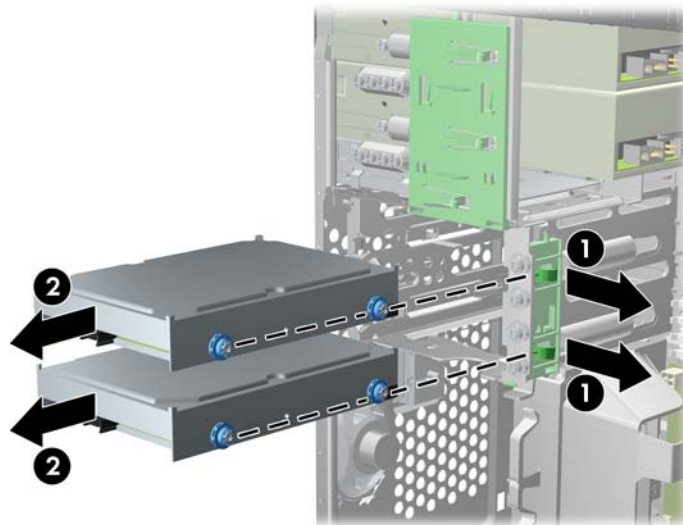
Figura 3-25 Extracción de una unidad de disco duro
