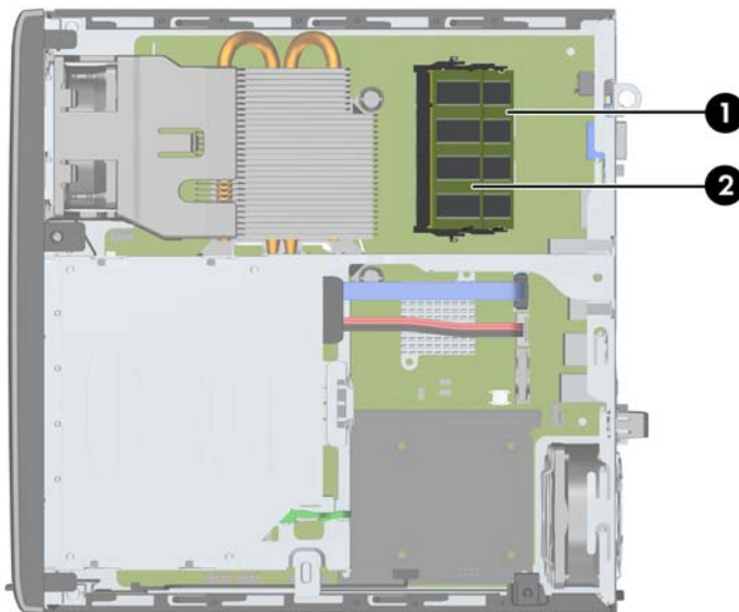
Figura 5-9 Ubicaciones de los sockets SODIMM
