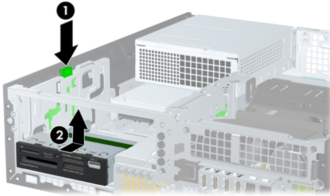
Figura 4-28 Extracción de una unidad de 3,5 pulgadas (se muestra el lector de tarjetas multimedia)
