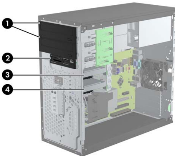
Figura 3-15 Posiciones de las unidades
