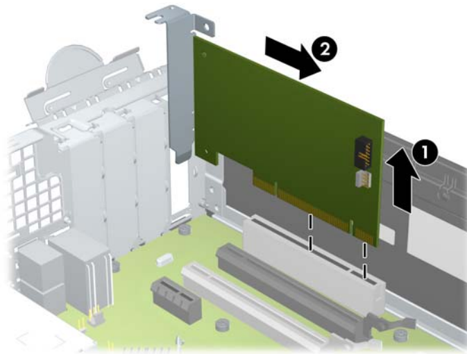
Figura 4-12 Extracción de la tarjeta de expansión PCI estándar
