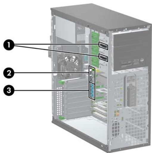
Figura 2-21 Ubicación de los tornillos guía adicionales
