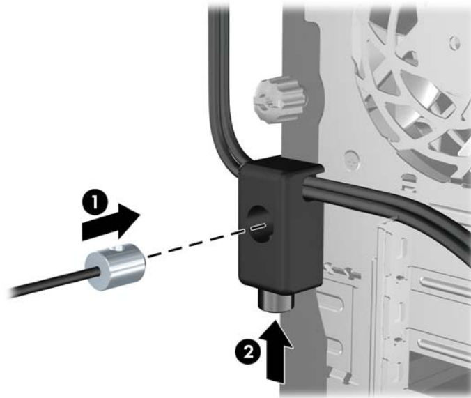
Figura 3-40 Activación del bloqueo
