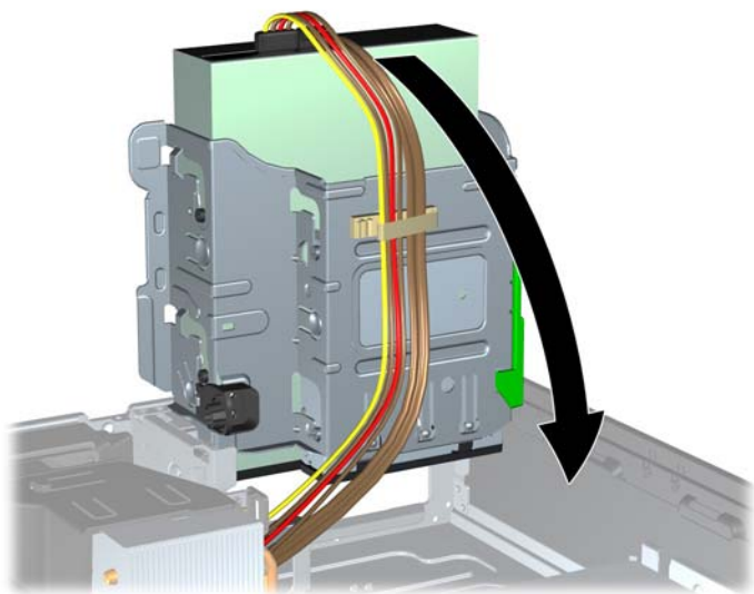
Figura 4-26 Giro del compartimiento para unidades hacia abajo
