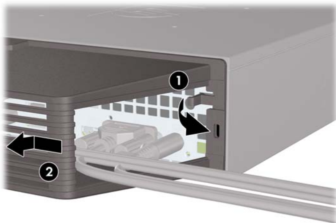
Figura 5-23 Extracción de una cubierta para puerto
