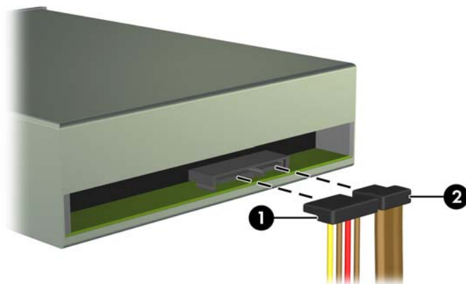
Figura 4-25 Conexión de los cables de alimentación y datos
