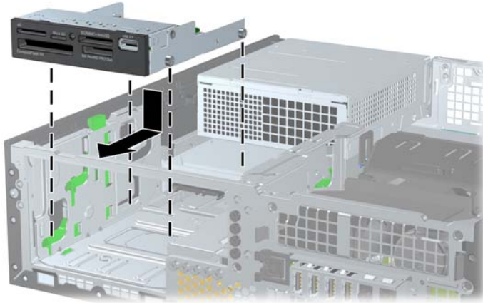
Figura 4-30 Instalación de una unidad en el compartimiento para unidades de 3,5 pulgadas (se muestra un lector de tarjetas multimedia)
