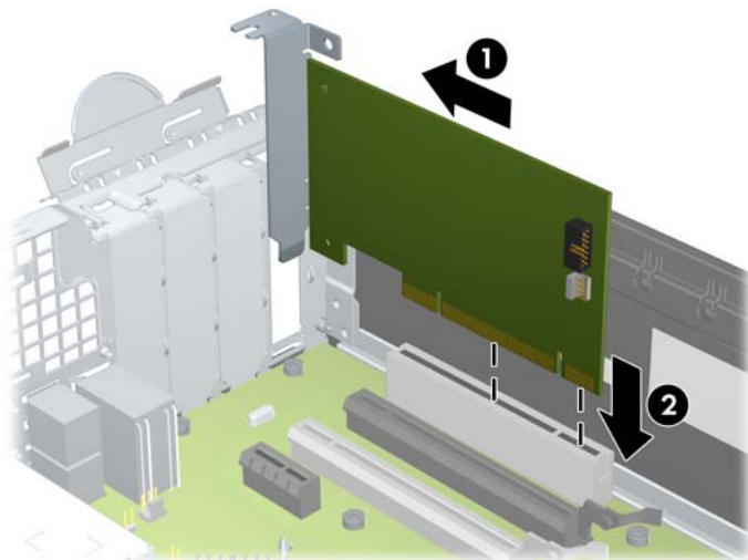
Figura 4-14 Instalación de una tarjeta de expansión
