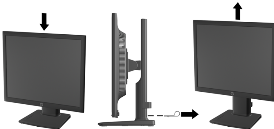
Abbildung 2-13 Lösen des Arretierstifts und Einstellen der Höhe (Modell HP LA1956x)
