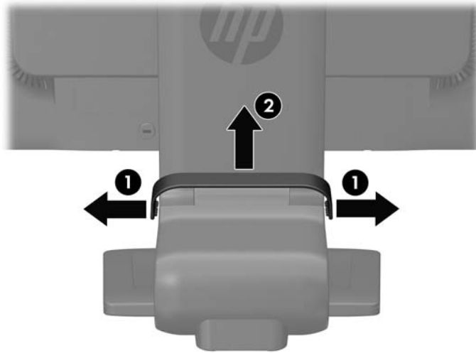
Abbildung 2-4 Entfernen des Kabelführungsclips (HP Modell LA1956x)
