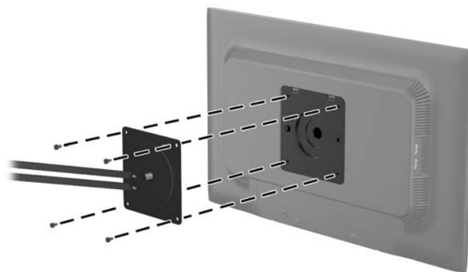
Abbildung 2-19 Montieren des Monitors
