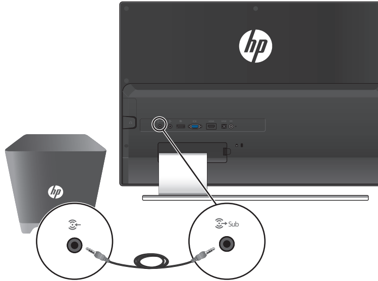
그림 3-5 서브우퍼 연결하기
