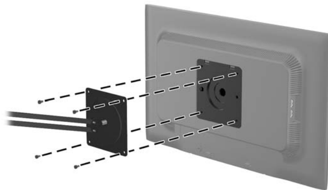
Figure 2-14 Montage du moniteur
