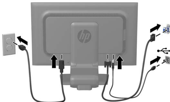
圖示 2-4 連接纜線
