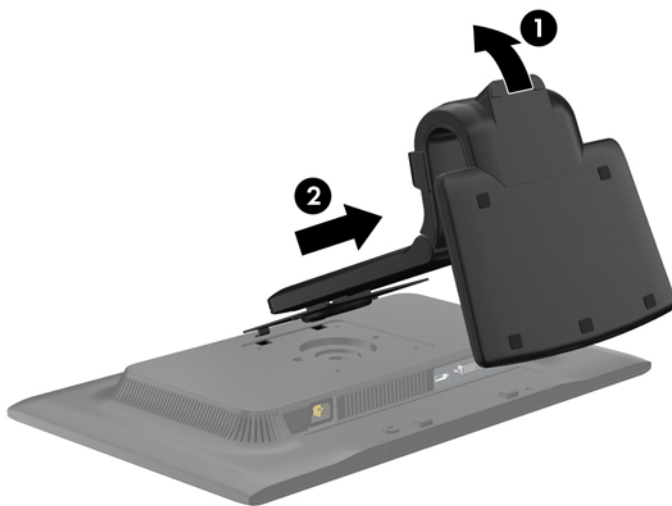
圖示 2-13 拆卸底座
