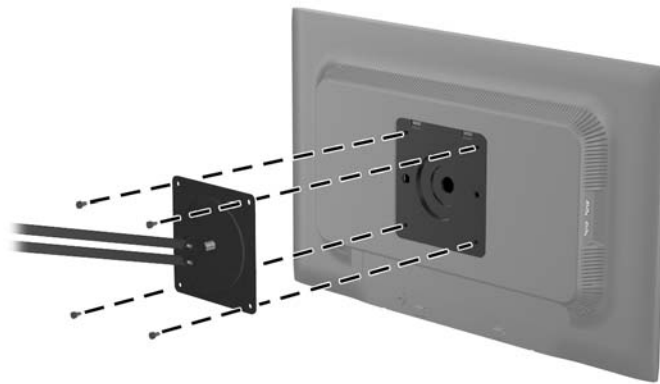
圖示 2-14 掛上顯示器
