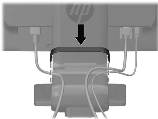
圖示 2-5 安裝纜線管理夾
