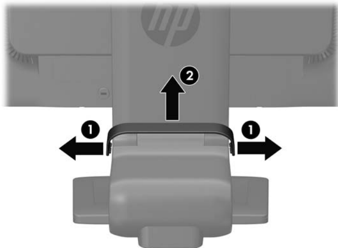
圖示 2-3 取下纜線管理夾
