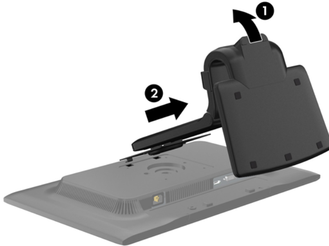
Figura 2-13 Extracción de la base del pedestal
