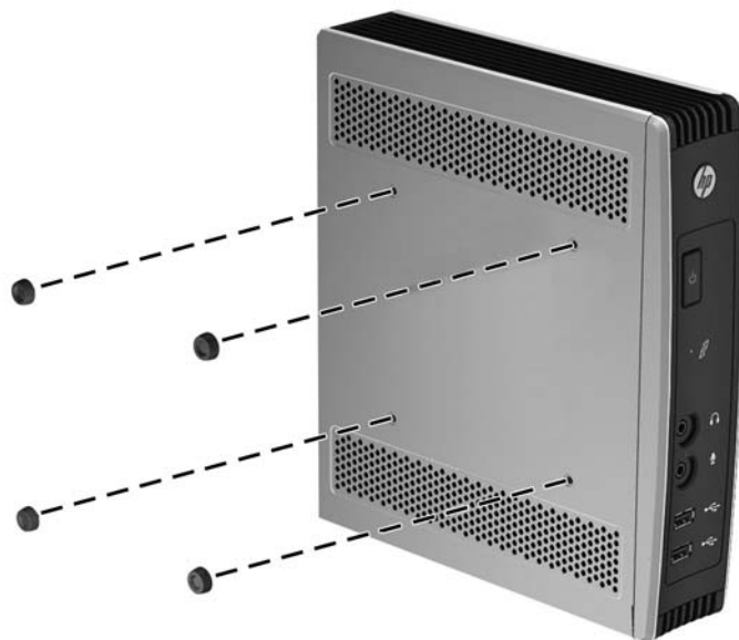
图 1-3 安装橡胶脚垫
