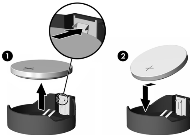
图 2-2 卸下并更换内置电池
