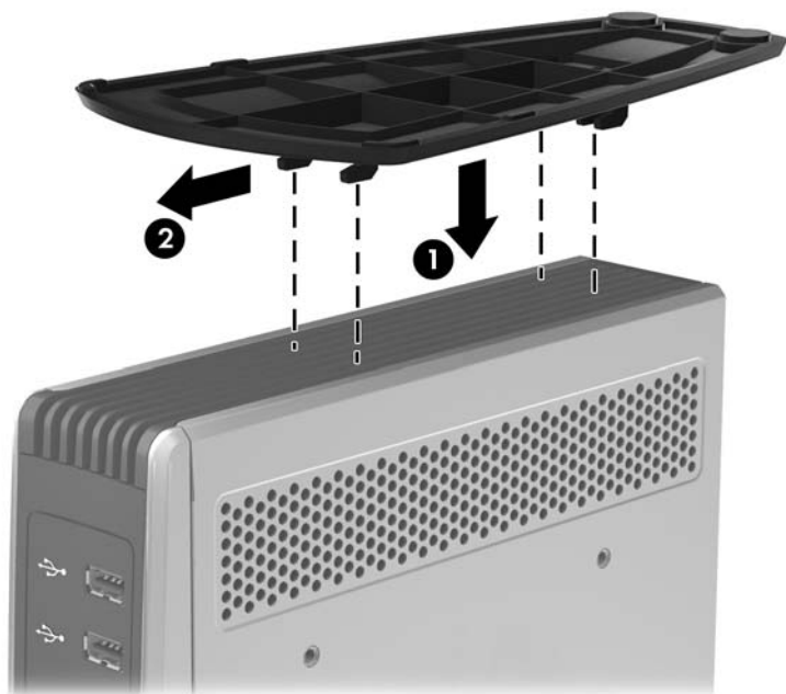
图 1-4 安装底座
