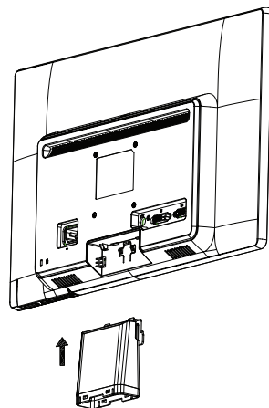
Figura 3-1 Colocación de la columna del monitor
