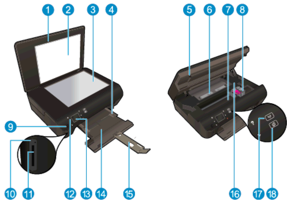
Рисунок 2-1 Вид HP ENVY 5530 e-All-in-One series спереди и сверху
